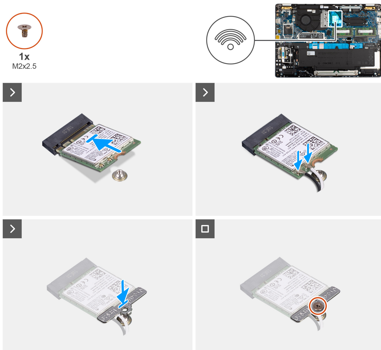
Figur 36. Installera WLAN-kortet
