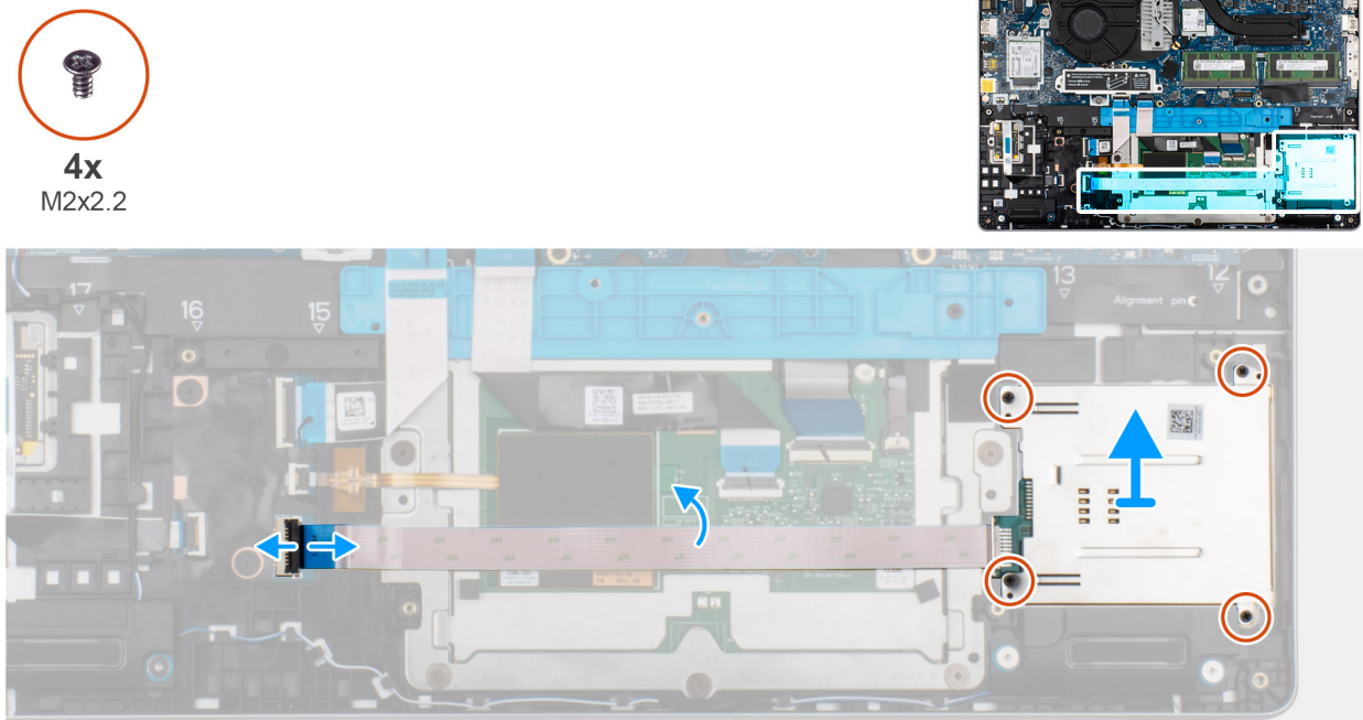
Figur 50. Ta bort smartkortläsaren
