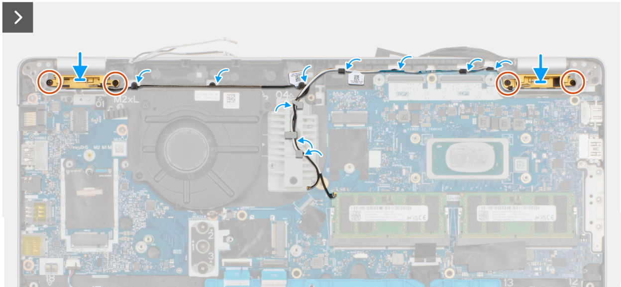
Figur 45. Installera WLAN-antennen
