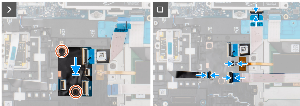
Figur 49. USH-kortet
