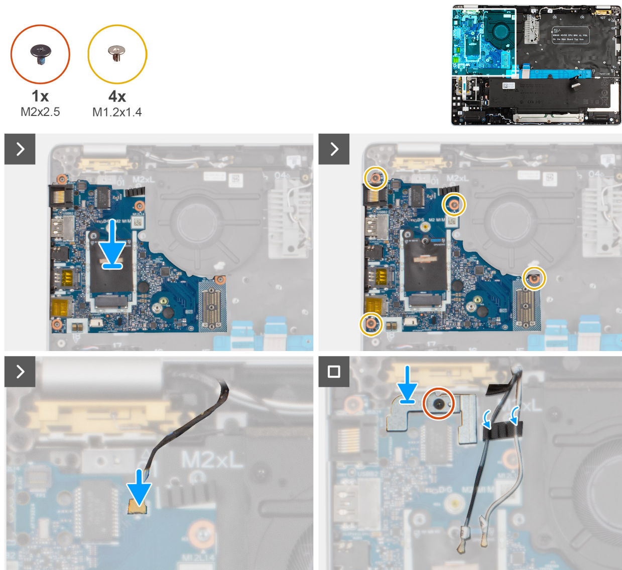
Figur 58. Ta bort I/O-kortet
