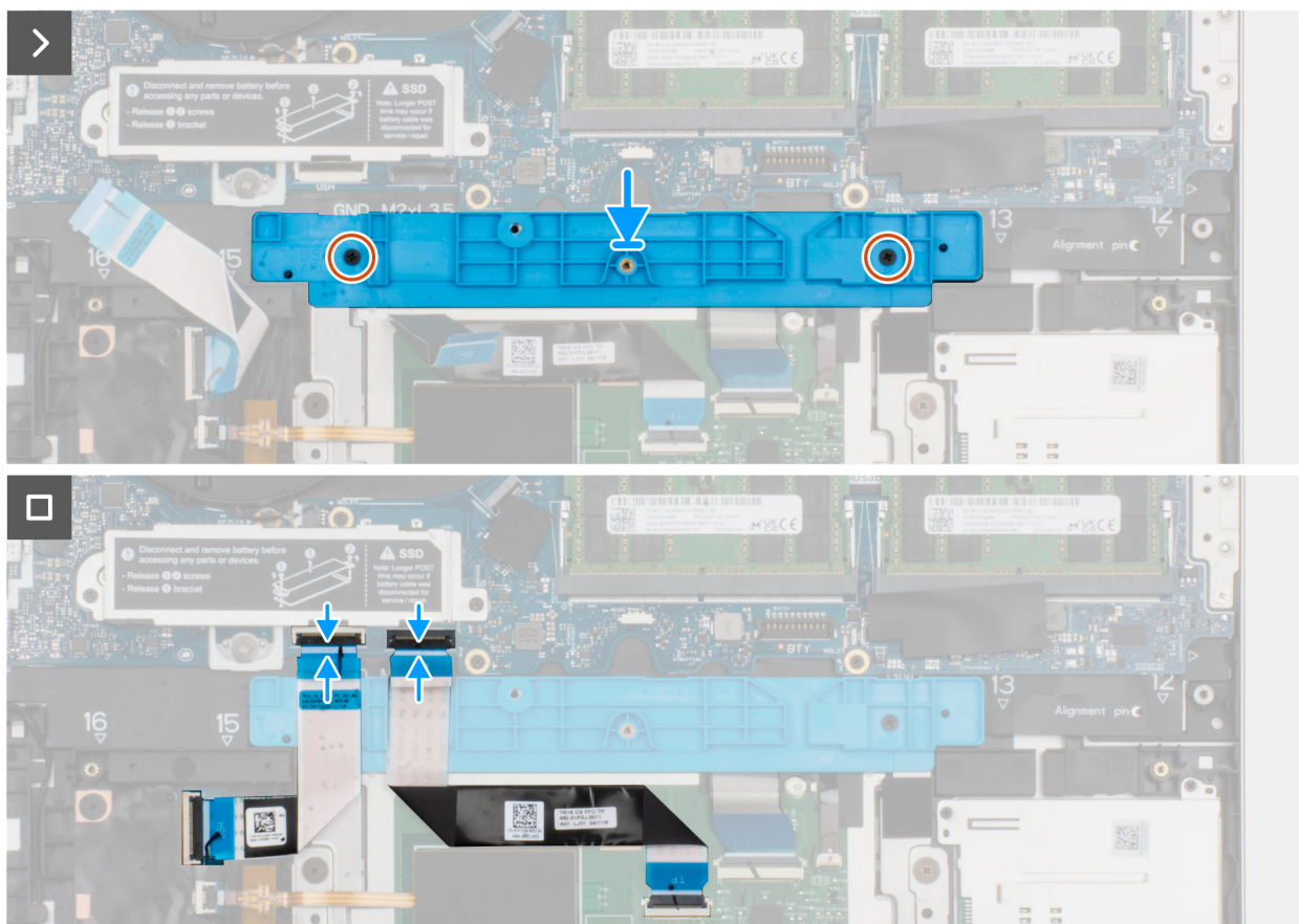
Figur 48. Installera batteristödkonsolen
