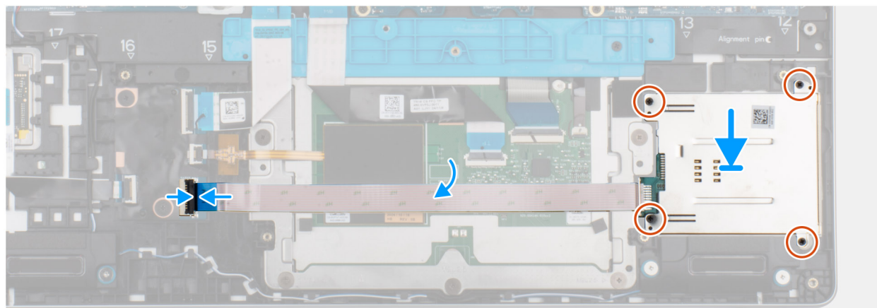
Figur 51. Installera smartkortläsaren
