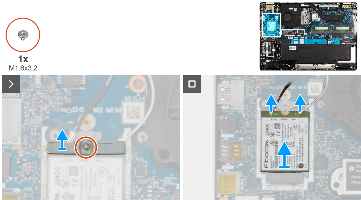
Figur 33. Ta bort 4G WWAN-kortet
