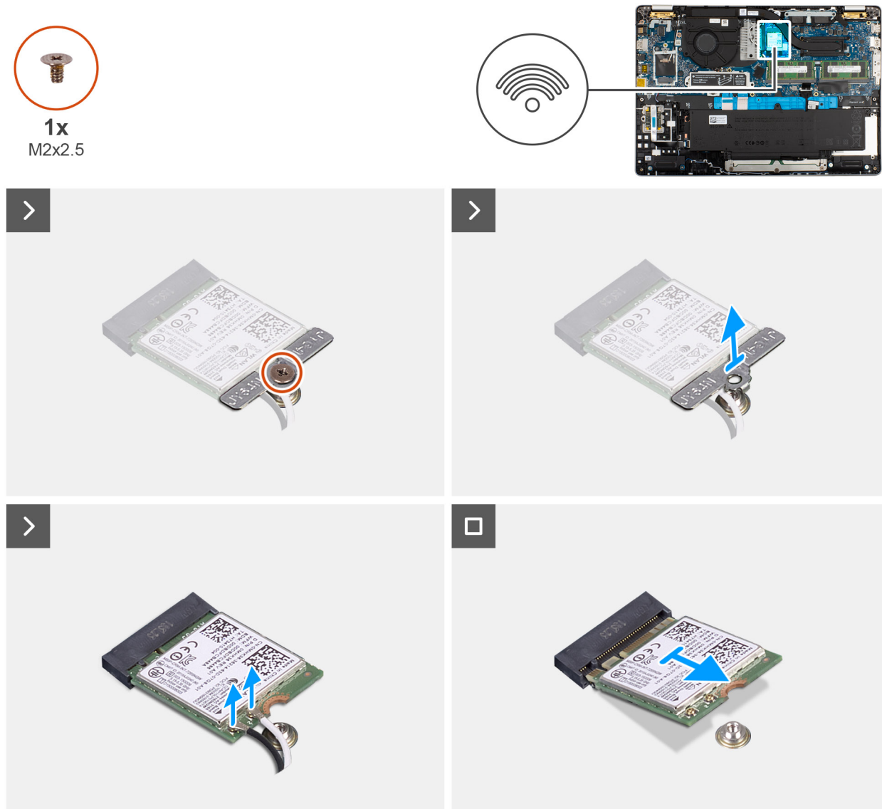
Figur 35. Ta bort WLAN-kortet
