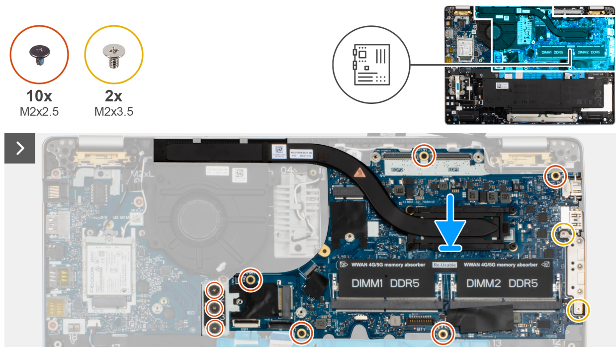
Figur 55. Installera moderkortet
