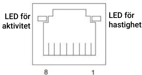
Figur 13. RJ45-port (kontaktsida)
