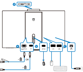
USB Type-C
