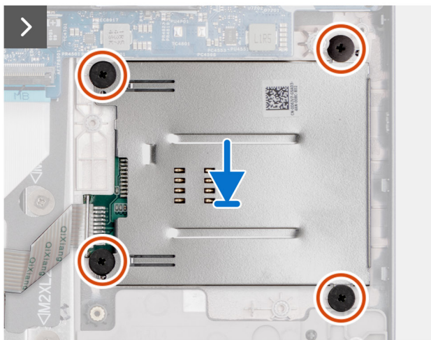
Figur 36. Installera smartkortläsaren
