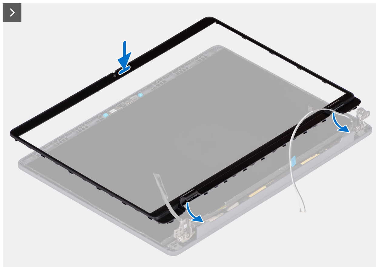
Figur 54. Installera bildskärmsramen
