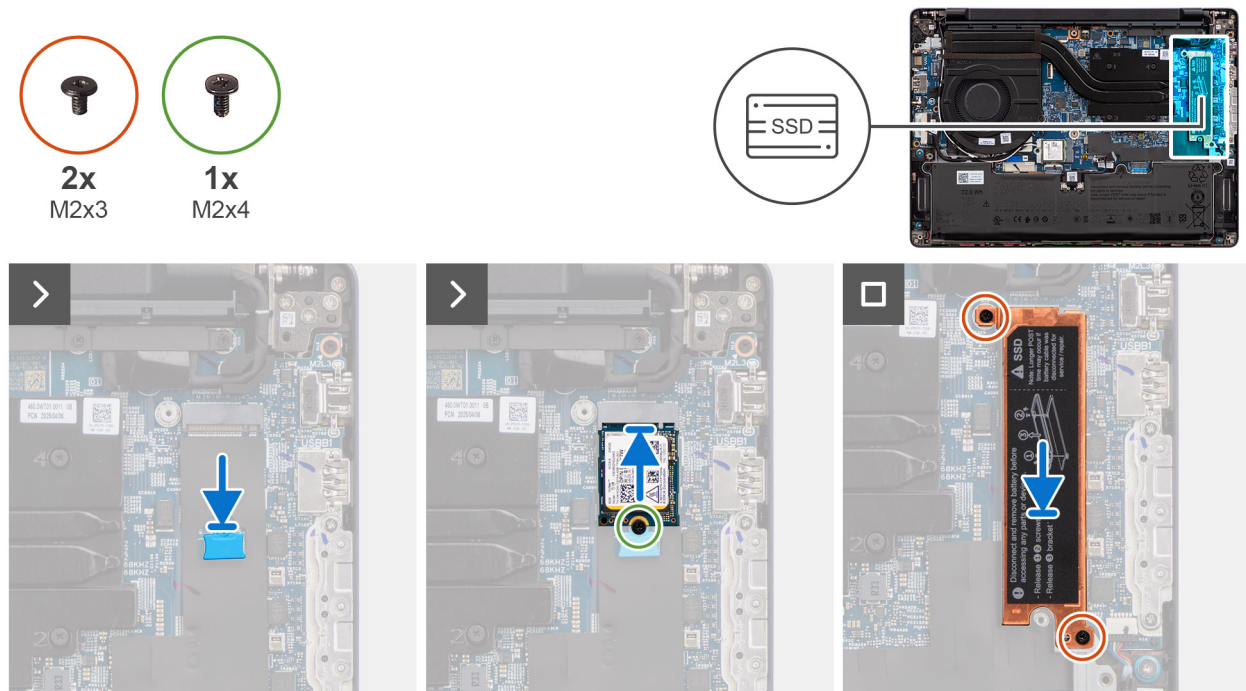
Figur 21. Installera M.2 2230 SSD-disken
