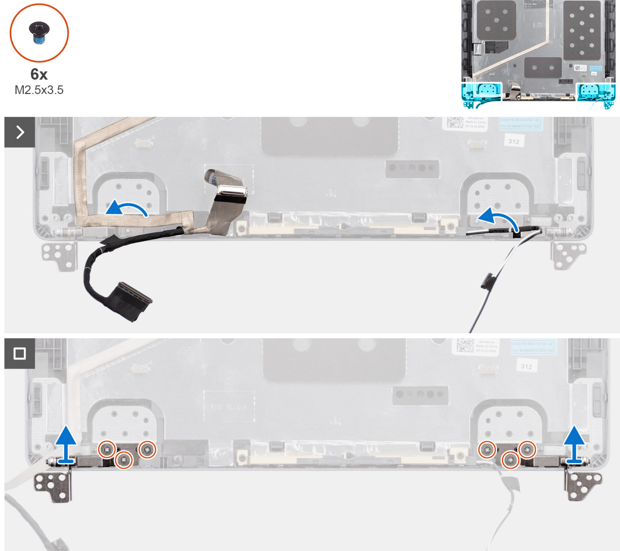
Figur 62. Ta bort bildskärmsgångjärnen
