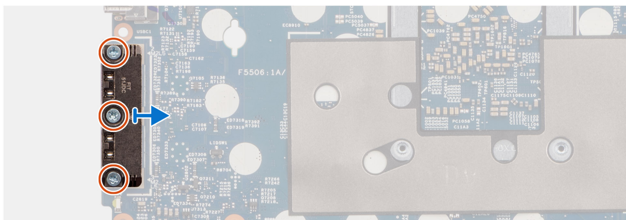
Figur 78. Ta bort USB Type-C-modulen
