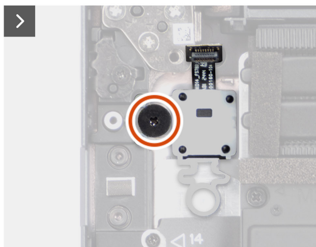
Figur 41. Ta bort strömbrytaren
