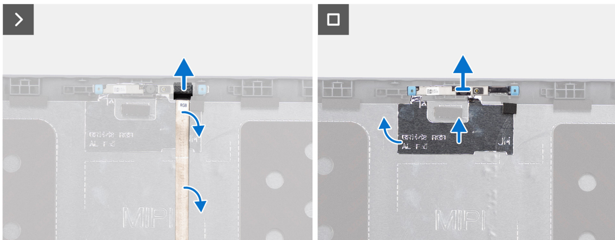
Figur 66. Ta bort kameran
