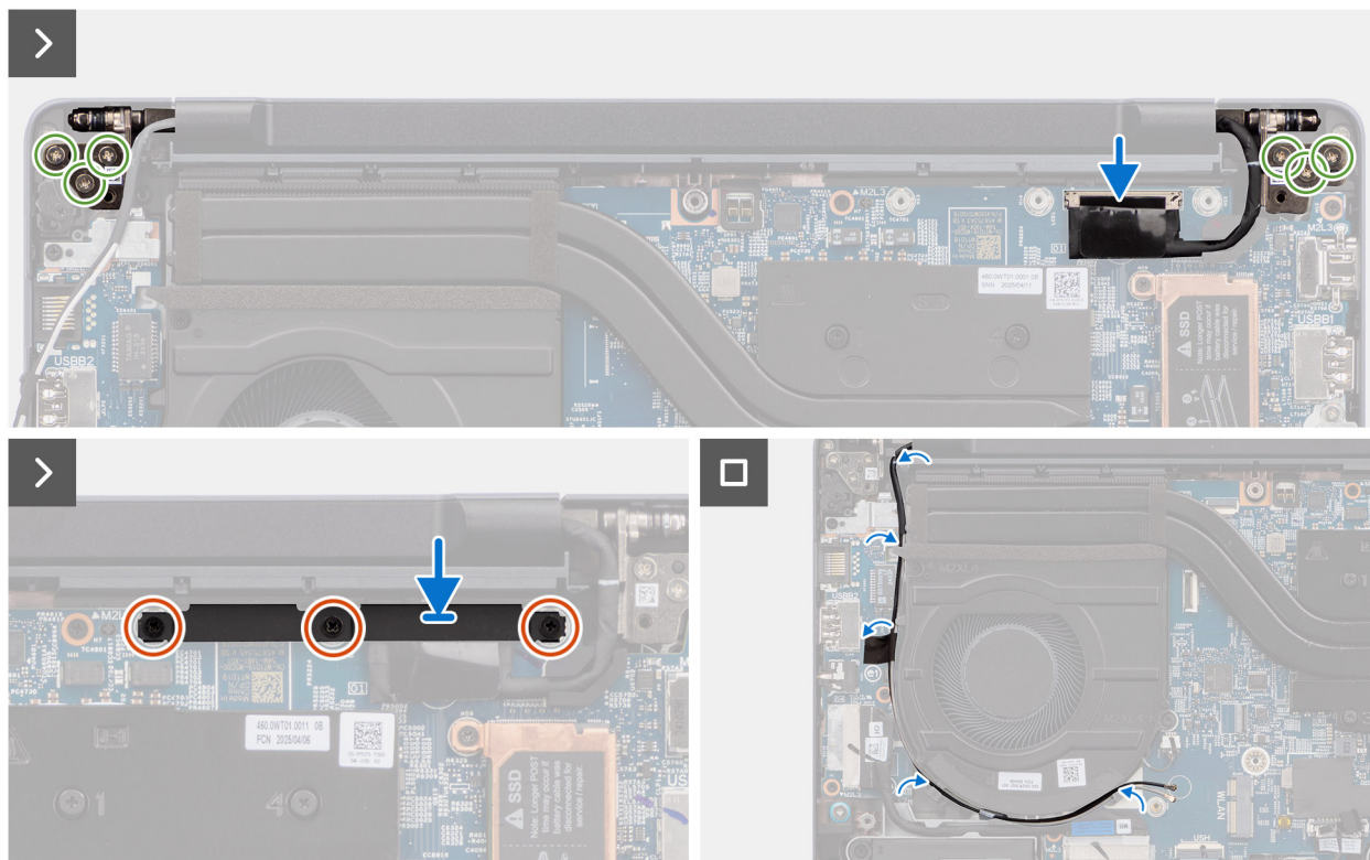
Figur 47. Installera bildskärmsenheten
