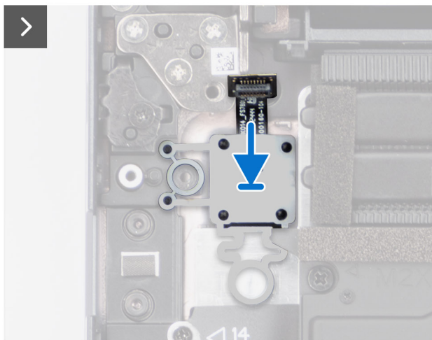
Figur 42. Installera strömbrytaren
