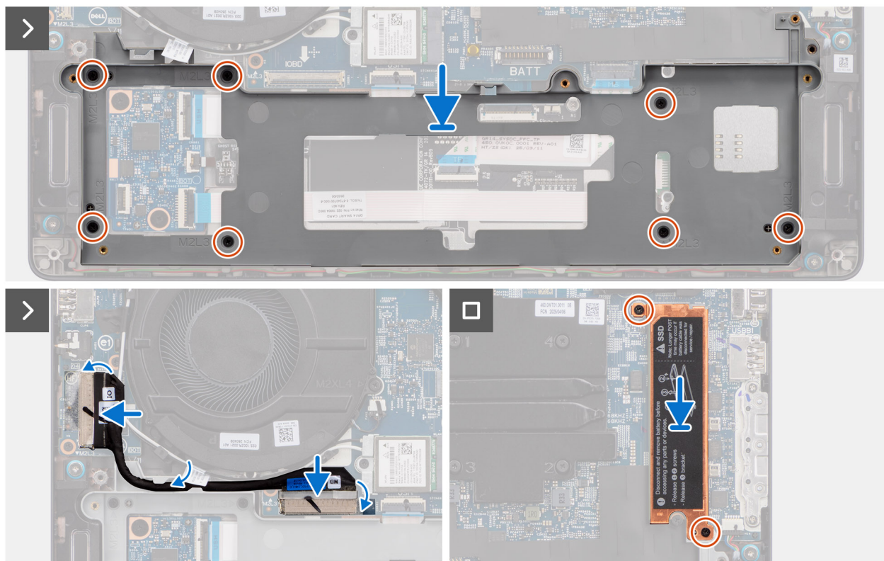
Figur 32. Installera batteriramen
