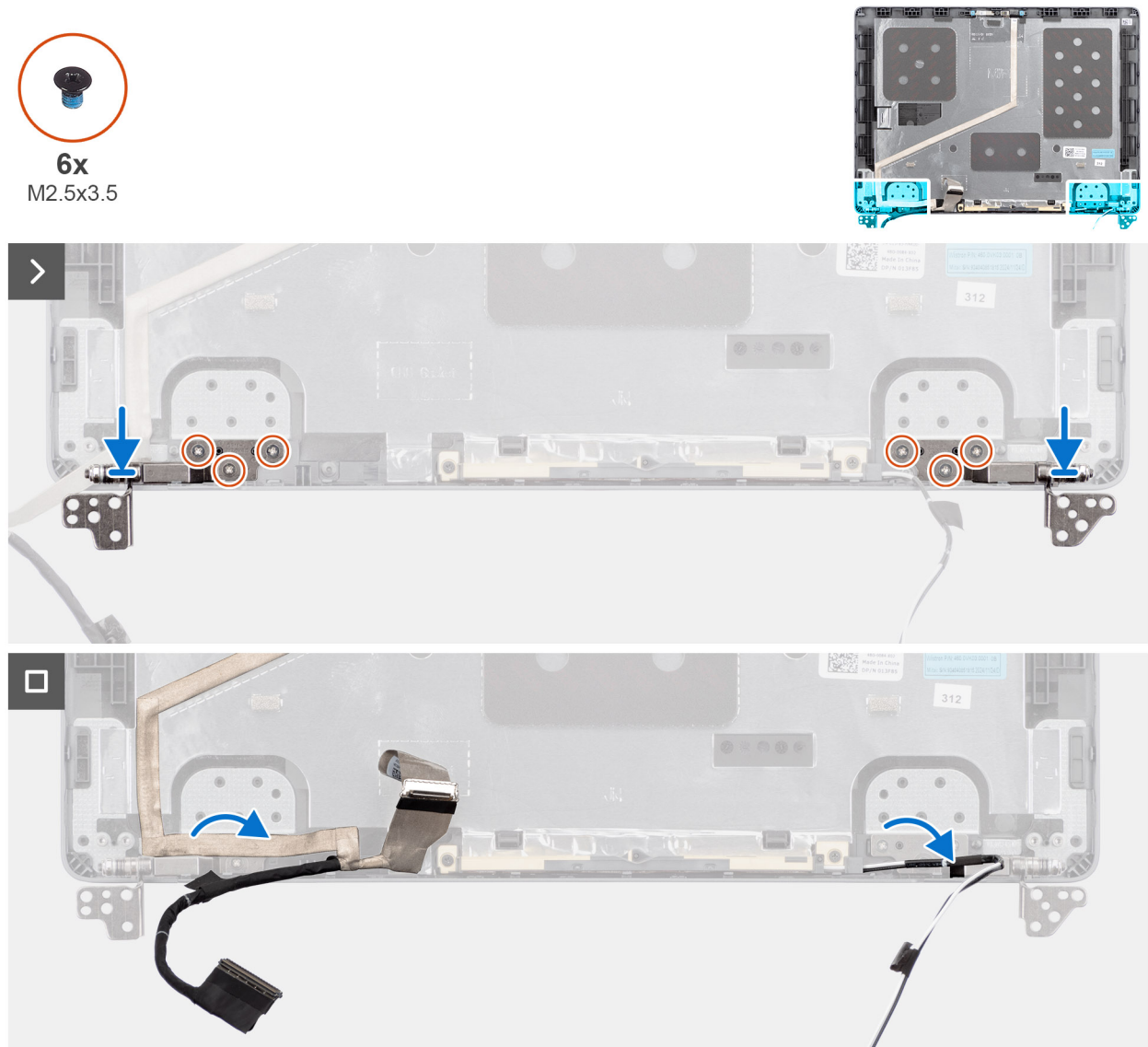
Figur 63. Installera bildskärmsgångjärnen
