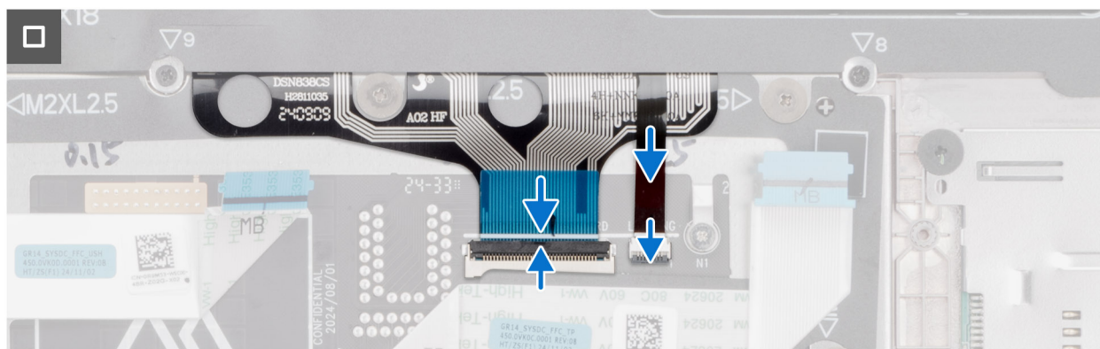
Figur 85. Installera tangentbordets kabel
