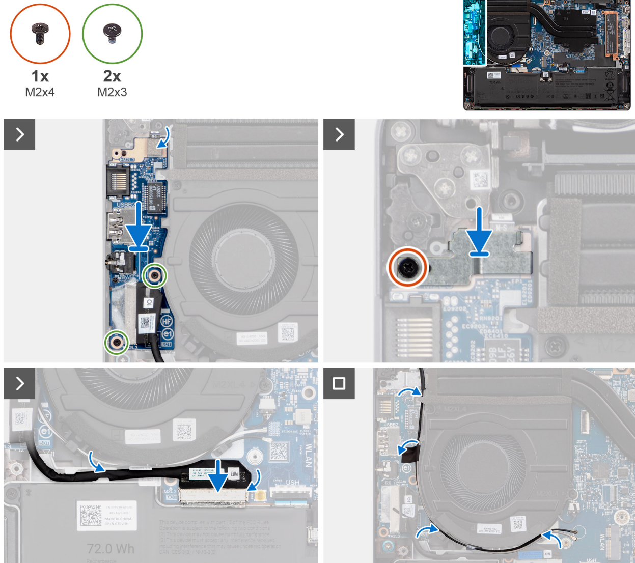
Figur 40. Installera I/O-kortet
