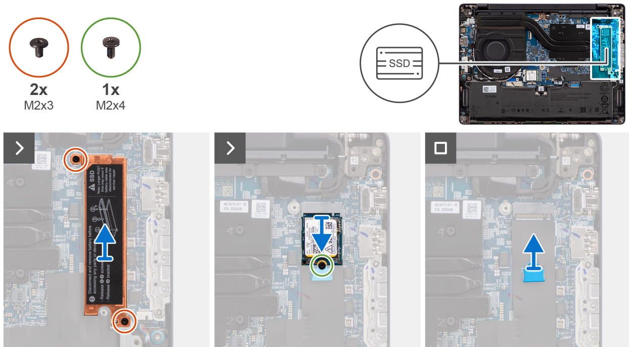
Figur 20. Ta bort M.2 2230 SSD-disken
