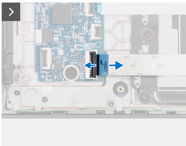
Figur 35. Ta bort smartkortläsaren
