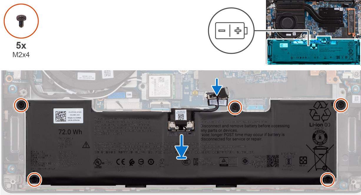
Figur 17. Installera batteriet
