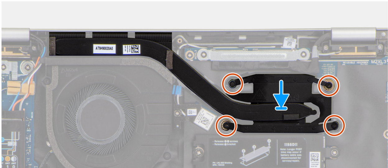
Figur 42. Installera kylflänsen
