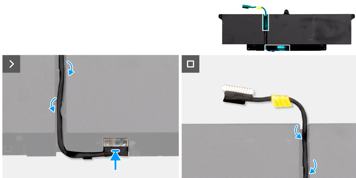
Figur 30. Installera batterikabeln
