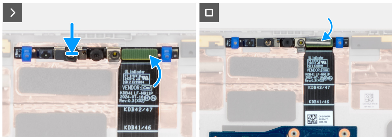
Figur 78. Installera MIPI-kameran
