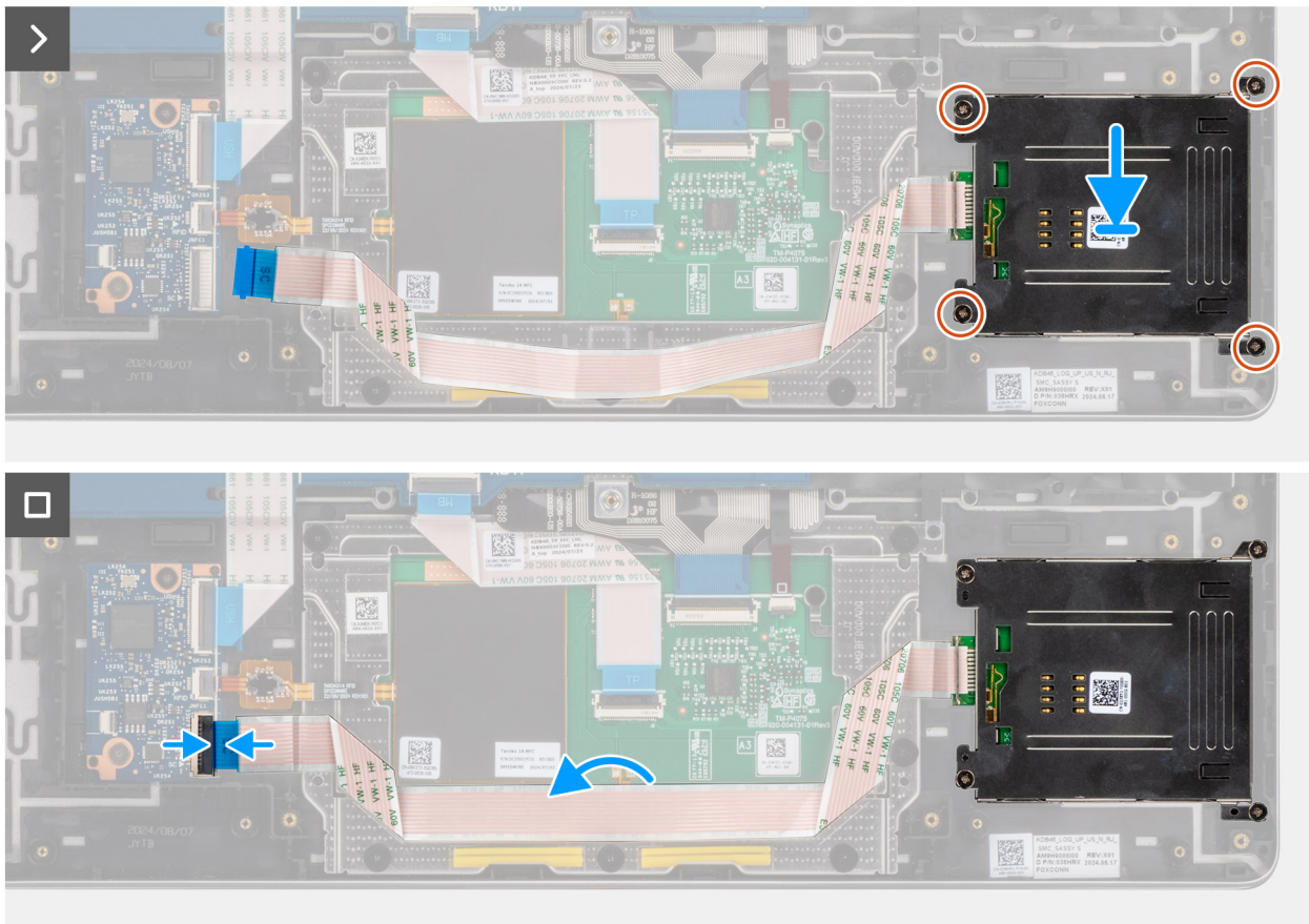
Figur 46. Installera smartkortläsaren
