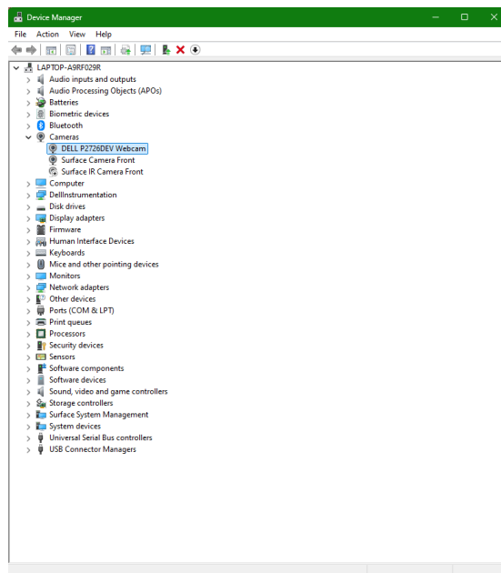
Figur 89. Enhetshanterarens gränssnitt.
