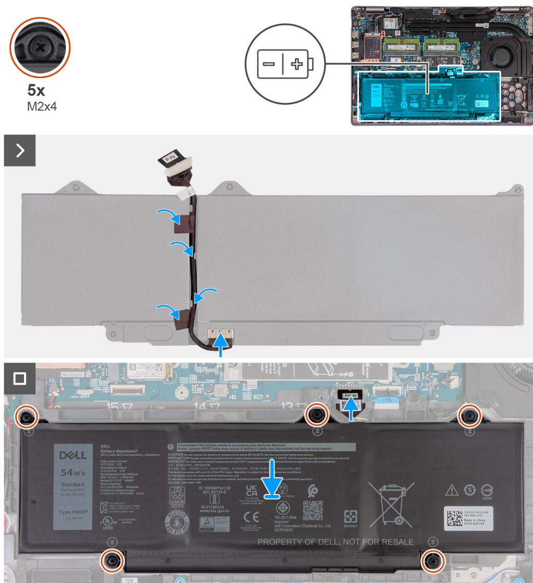
Figur 36. Installera batteriet
