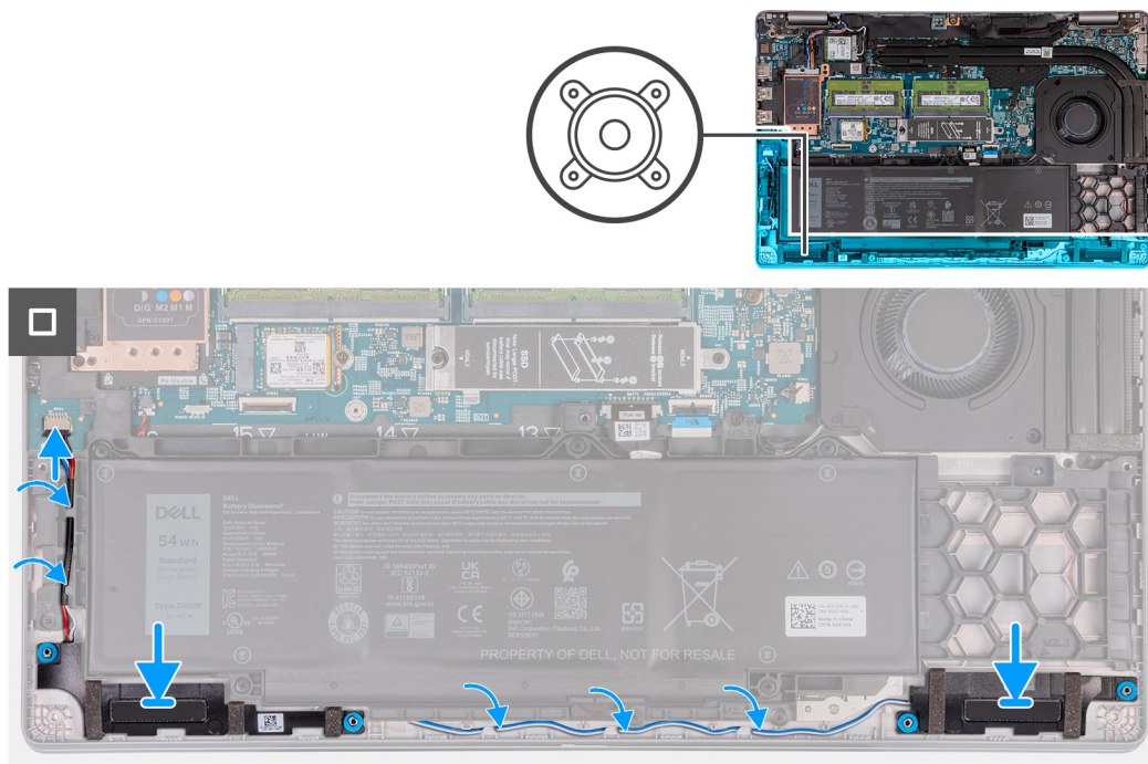
Figur 44. Installera högtalarna
