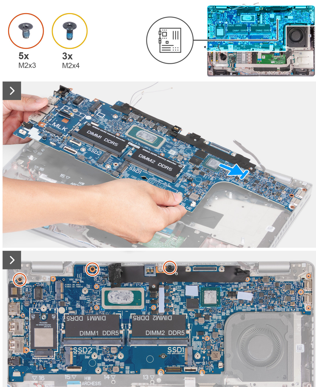
Figur 58. Installera moderkortet
