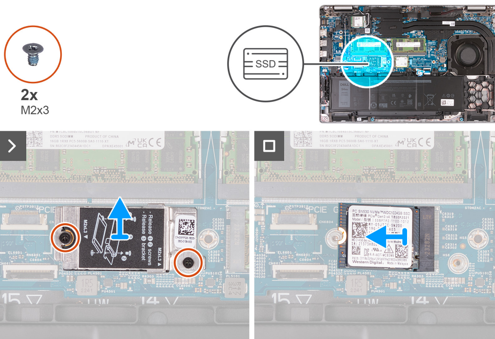
Figur 31. Ta bort M.2 2230 SSD-disk från kortplats 2
