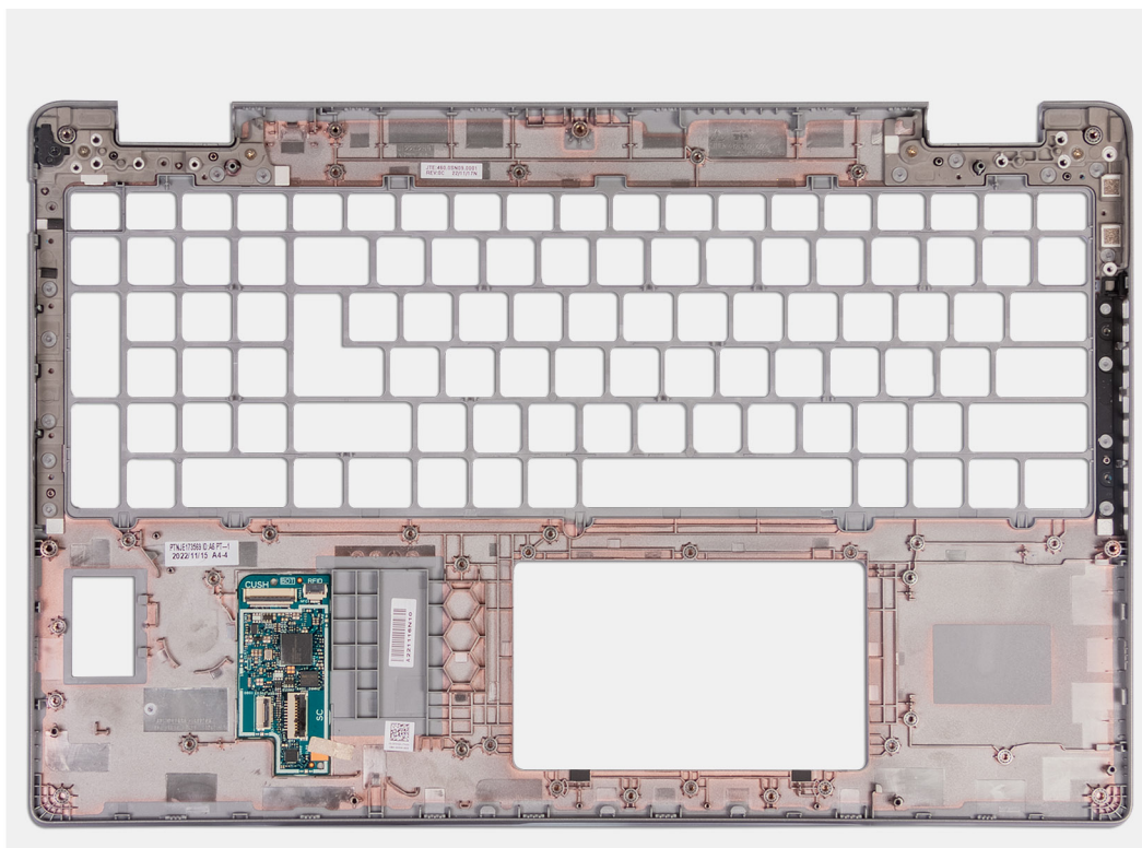
Figur 100. Ta bort handledsstödet
