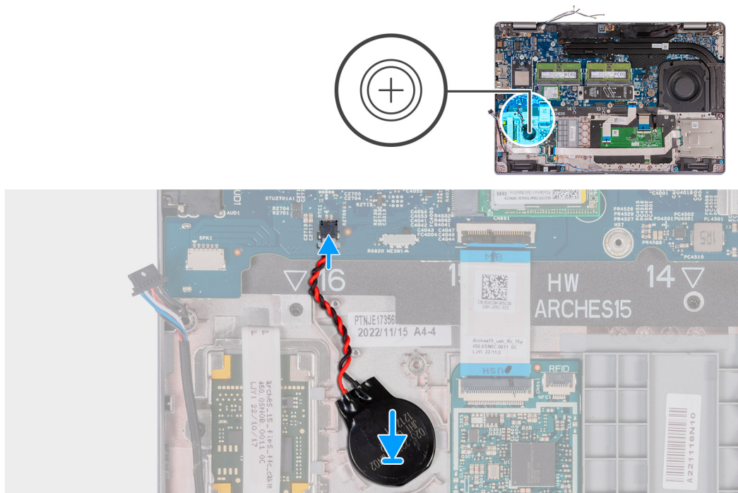
Figur 47. Installera knappcellsbatteriet
