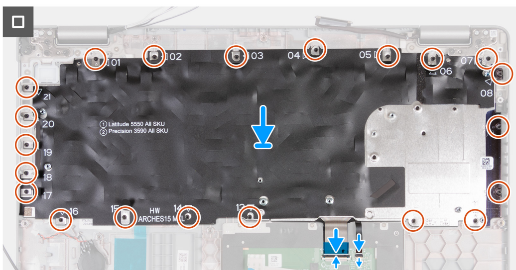
Figur 68. Installera tangentbordet
