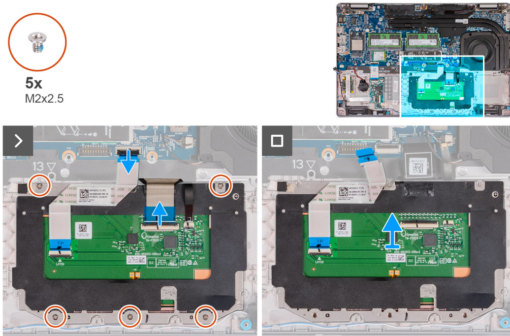
Figur 41. Ta bort styrplattan
