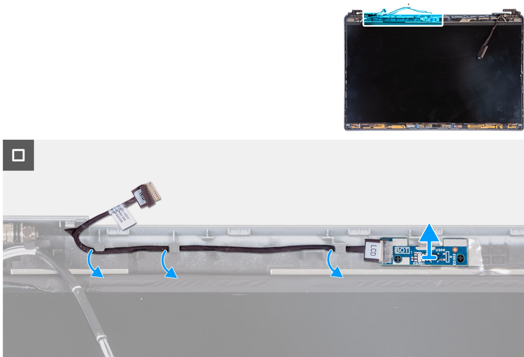
Figur 92. Ta bort sensorkortet
