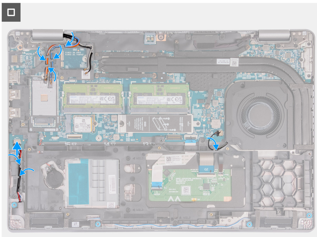
Figur 40. Dra kablarna
