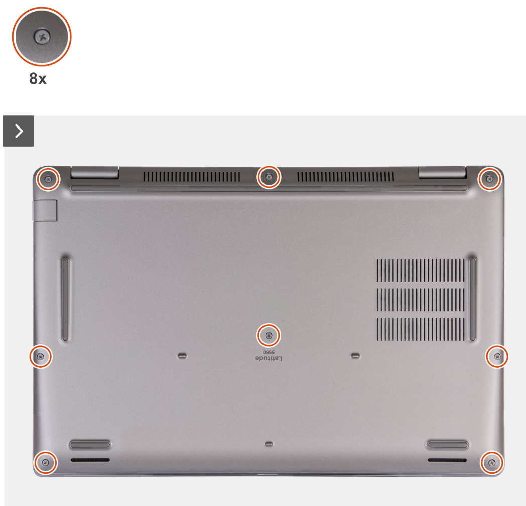
Figur 13. Lossa fästskruvarna
