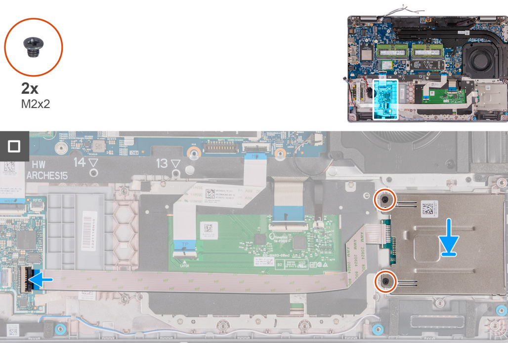
Figur 97. Installera smartkortläsaren
