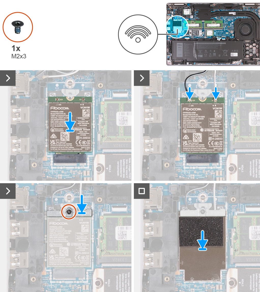
Figur 22. Installera 4G WWAN-kortet
