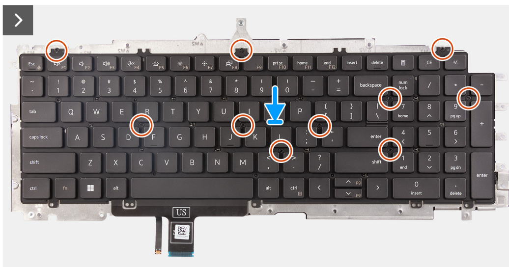
Figur 67. Installera tangentbordet
