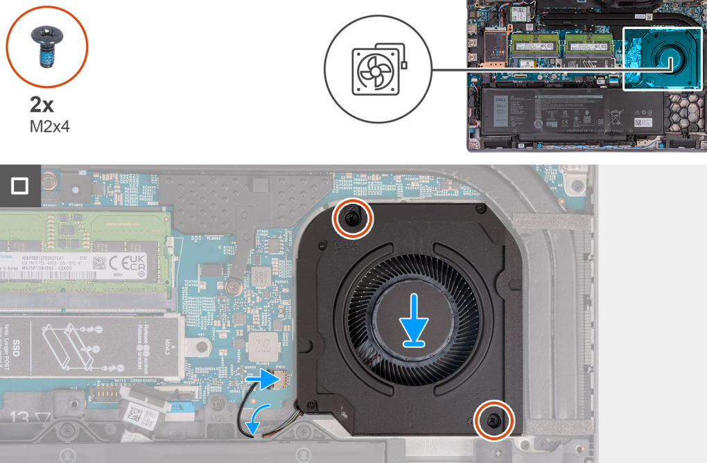
Figur 34. Installera fläkten
