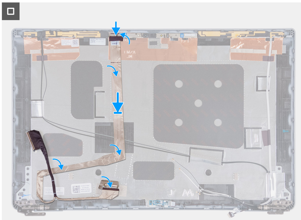
Figur 91. Installera bildskärmskabeln
