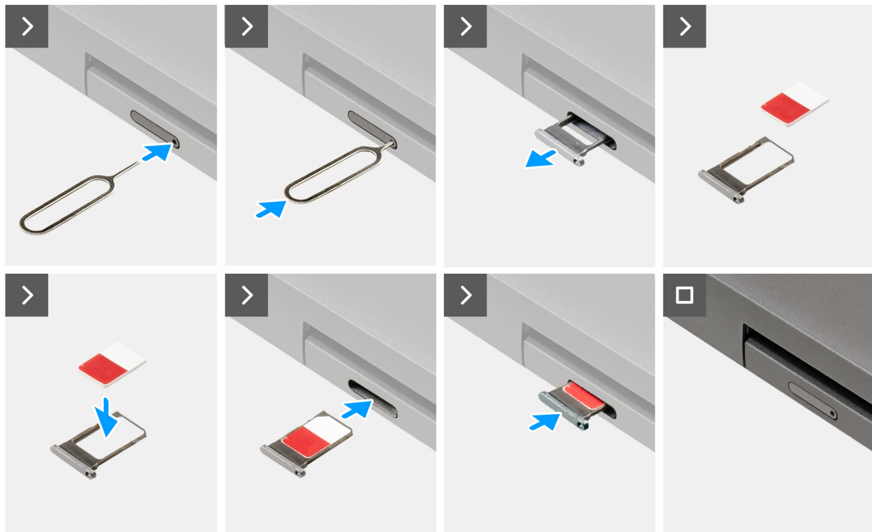
Figur 12. Installera SIM-kortfacket
