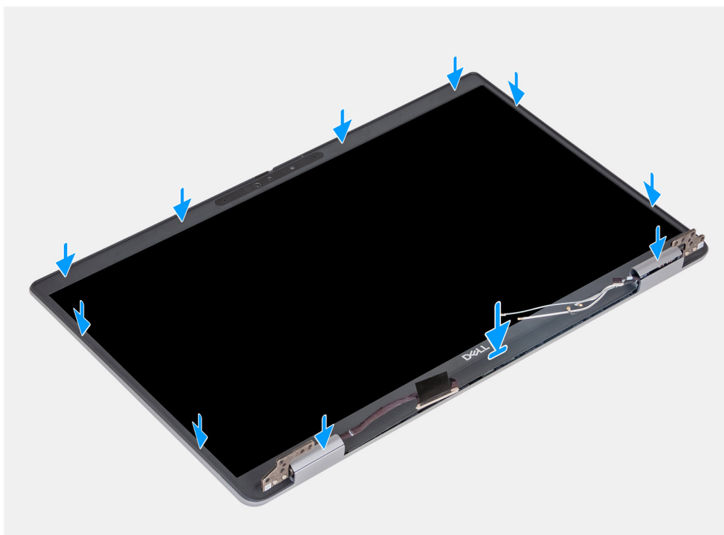
Figur 75. Installera bildskärmsramen
