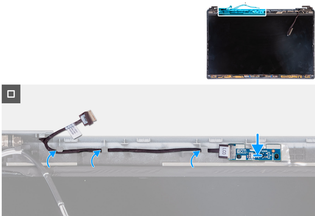
Figur 93. Installera sensorkortet
