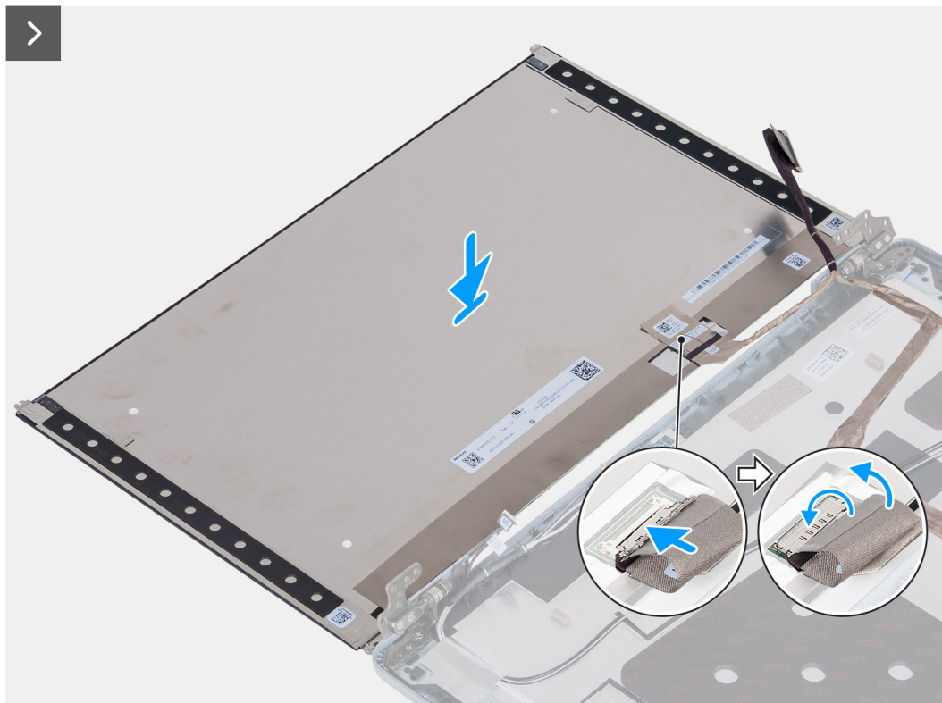
Figur 81. Installera bildskärmen
