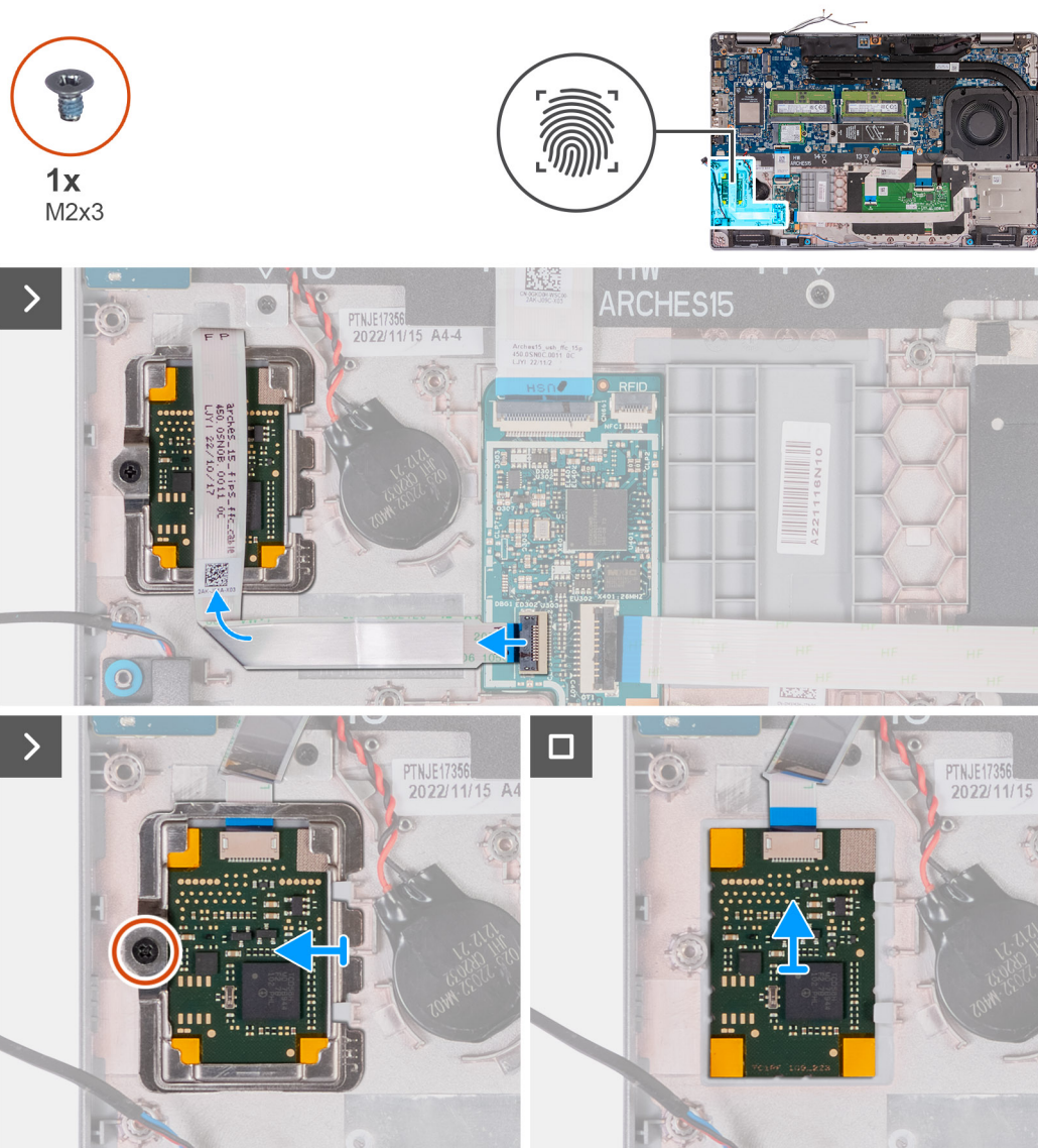
Figur 94. Ta bort fingeravtrycksläsaren
