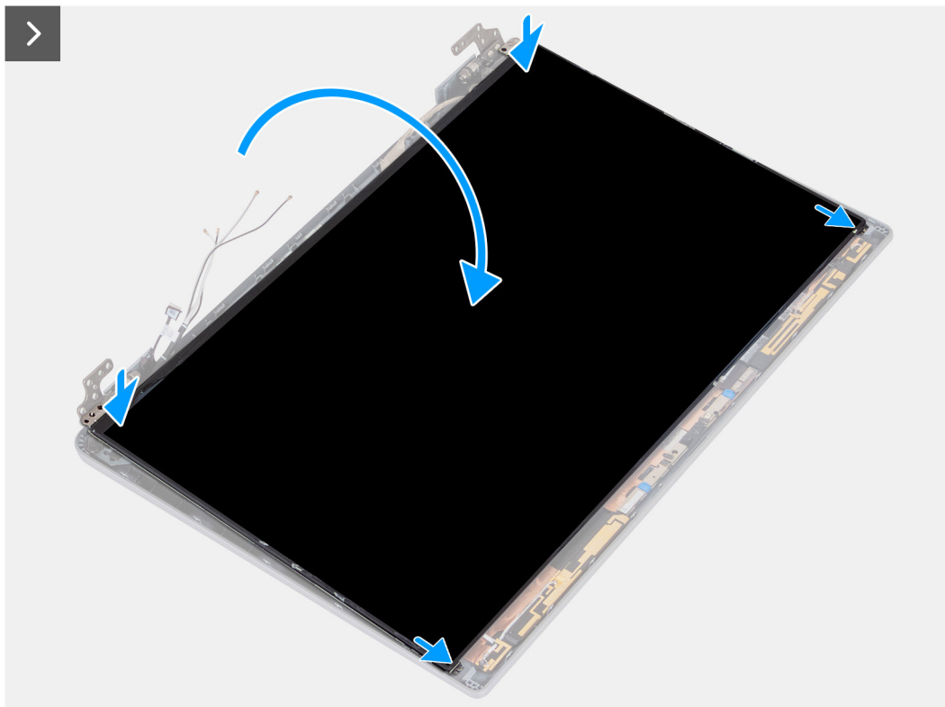
Figur 82. Installera bildskärmen
