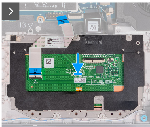
Figur 42. Installera styrplattan
