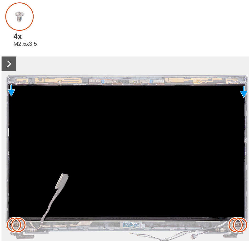
Figur 76. Ta bort bildskärmen
