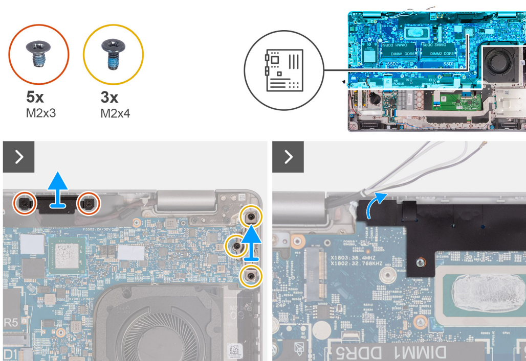
Figur 53. Ta bort skruvarna
