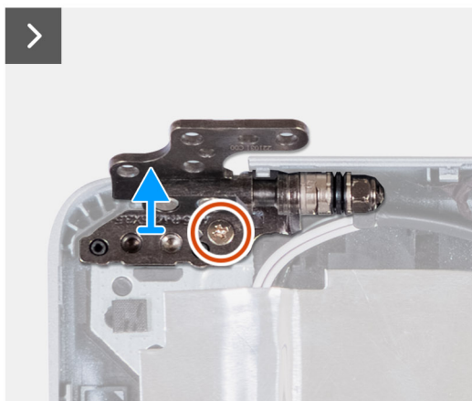
Figur 86. Ta bort bildskärmsgångjärnen
