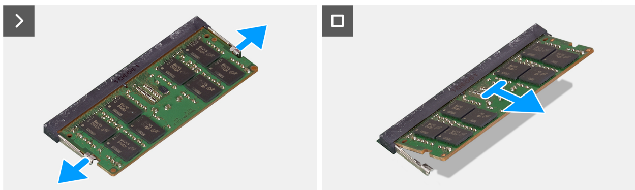
Figur 21. Ta bort minnesmodulen
