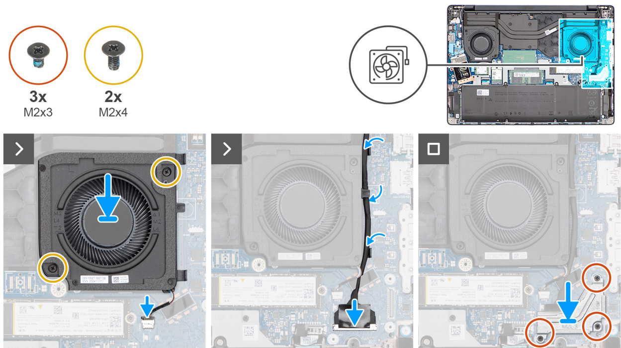
Figur 39. Installera den vänstra videofläkten/videofläkten
