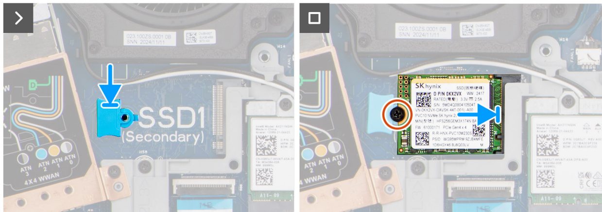
Figur 24. Installera M.2 2230 SSD-disken
