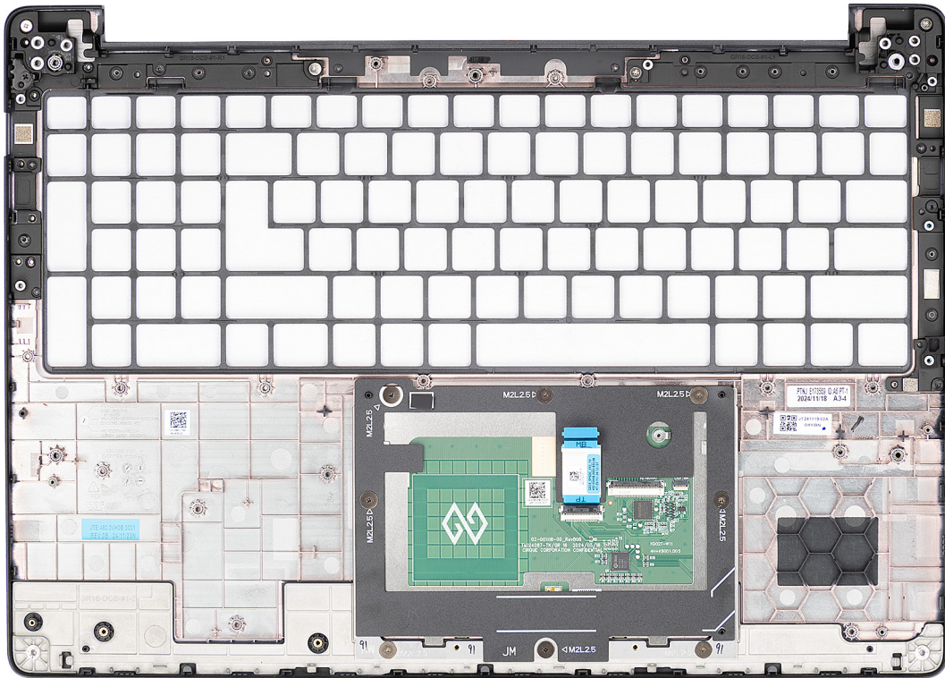
Figur 102. Handledsstöd
