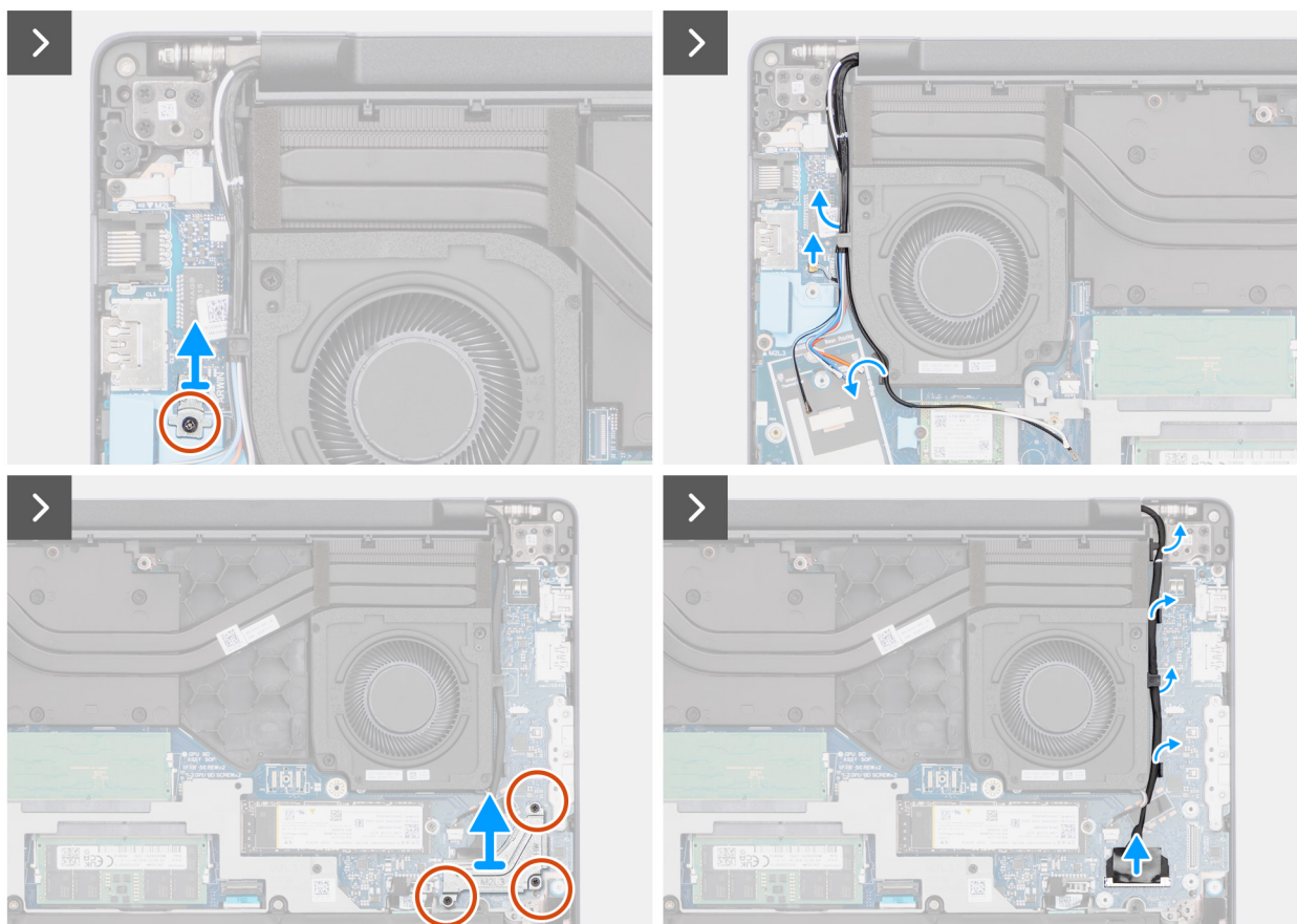
Figur 54. Ta bort bildskärmsenheten
