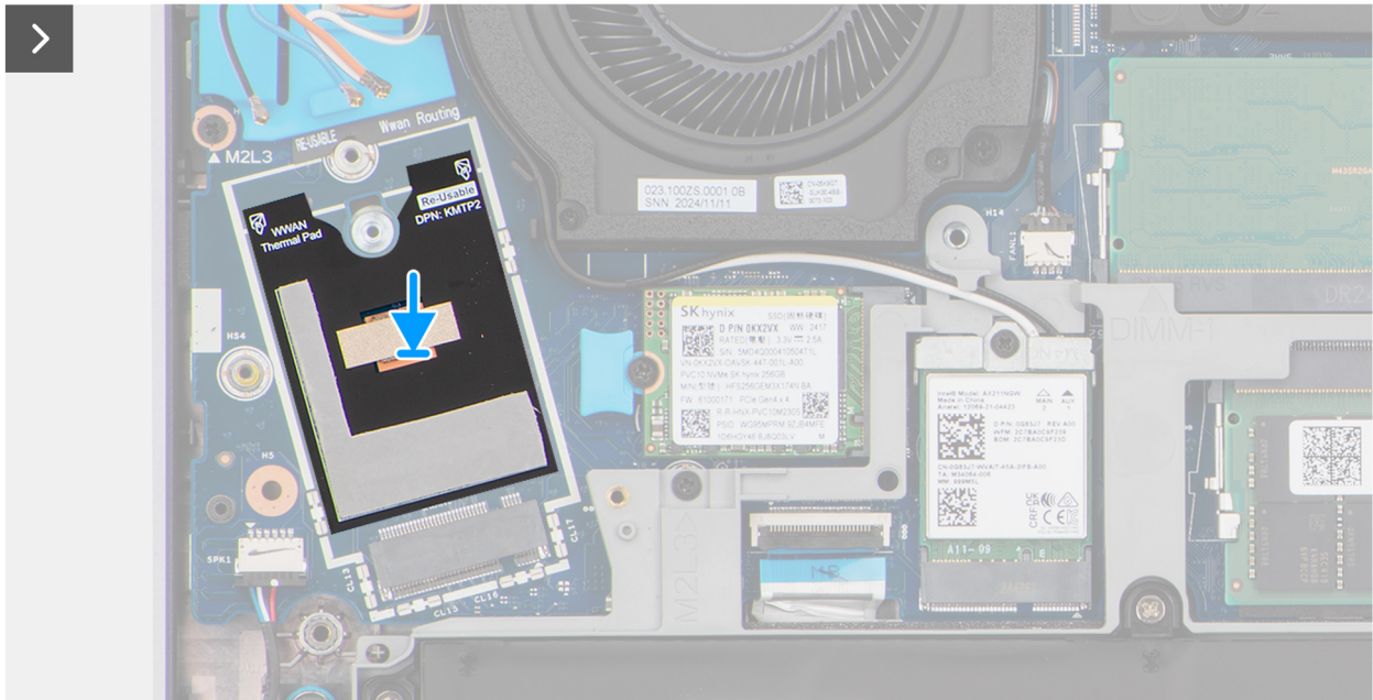
Figur 31. Installera WWAN-modulen
