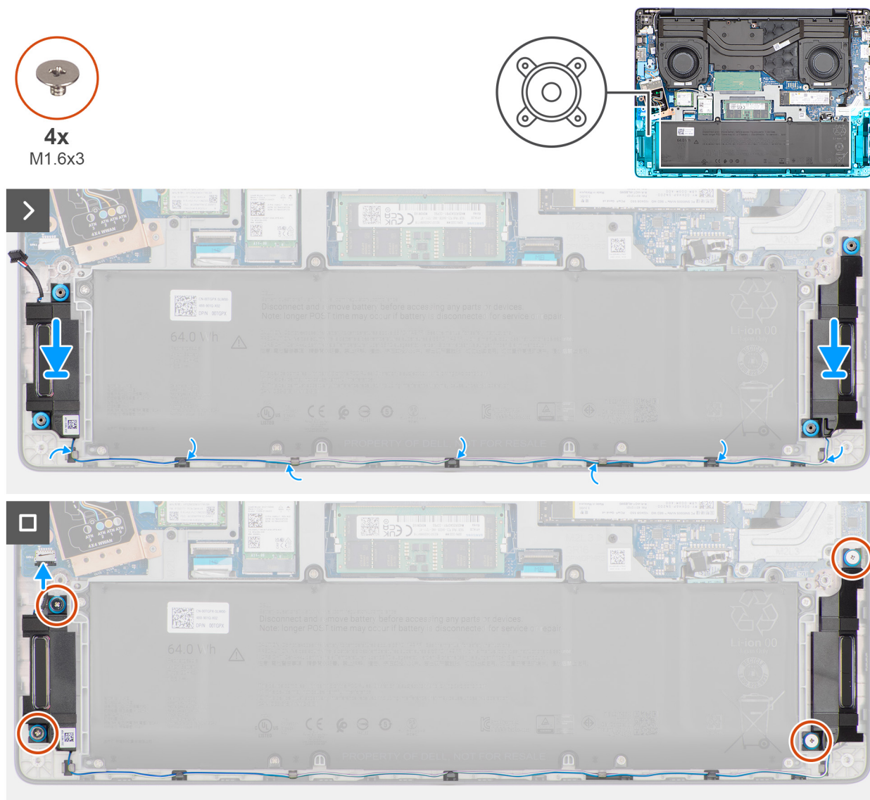
Figur 34. Installera högtalarna
