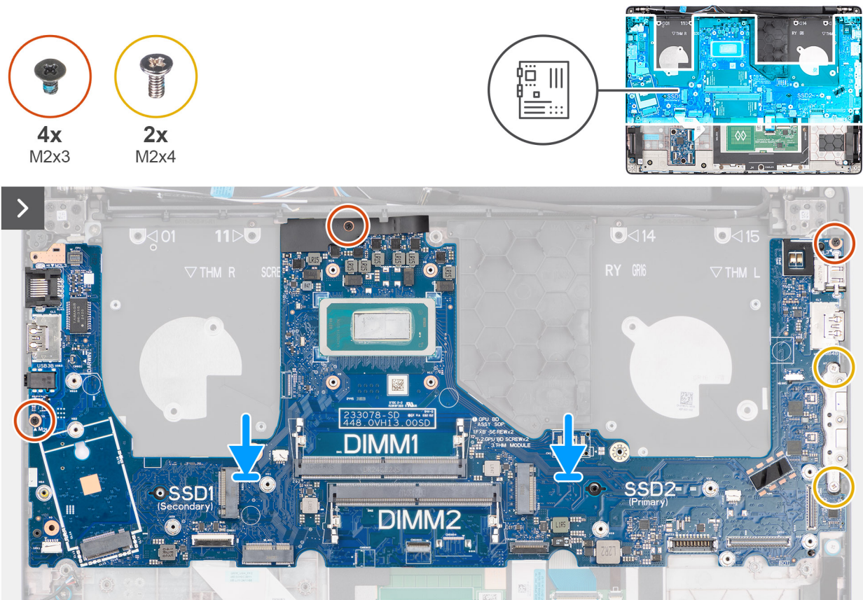
Figur 86. Installera moderkortet
