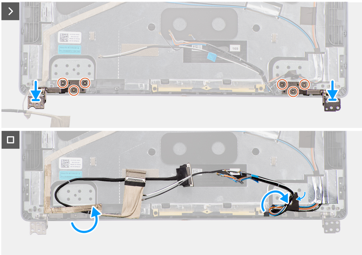
Figur 75. Installera bildskärmsgångjärnen
