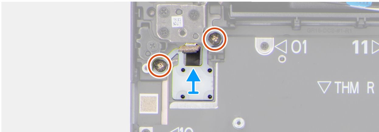
Figur 96. Ta bort strömbrytaren
