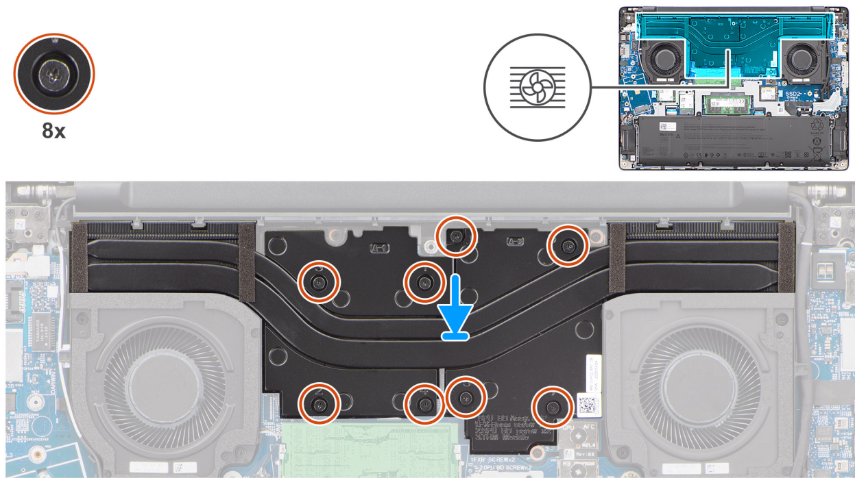
Figur 43. Installera kylflänsen
