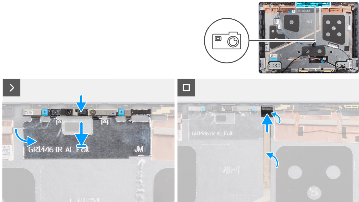
Figur 79. Installera kameran
