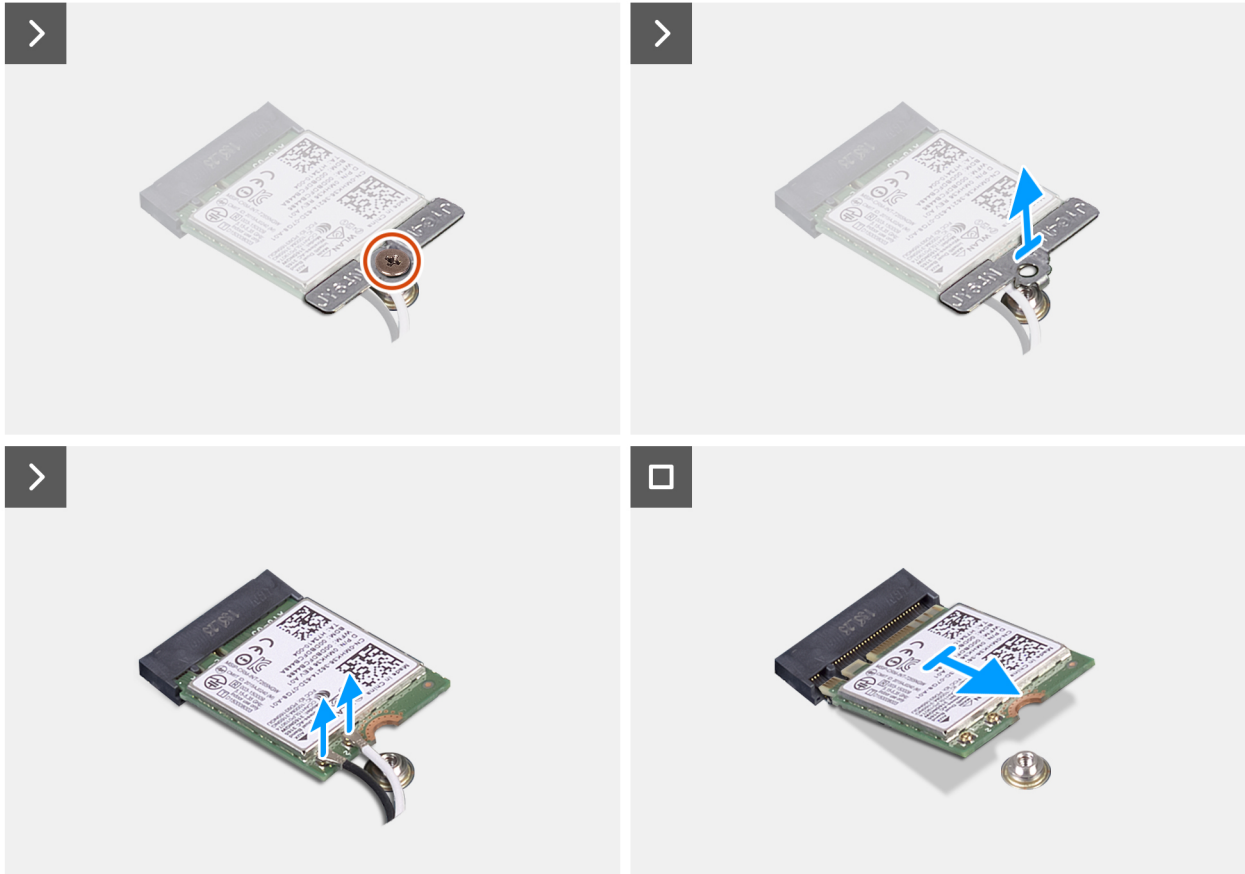
Figur 27. Ta bort det trådlösa kortet
