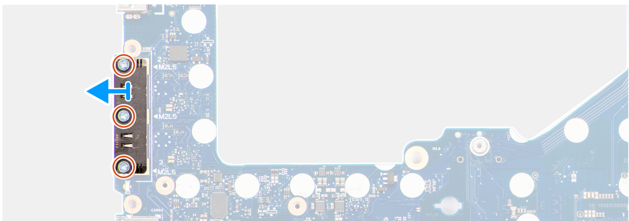
Figur 94. Ta bort USB Type-C-modulen
