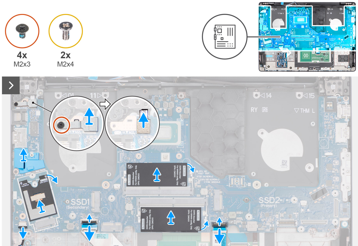
Figur 83. Ta bort systemkort
