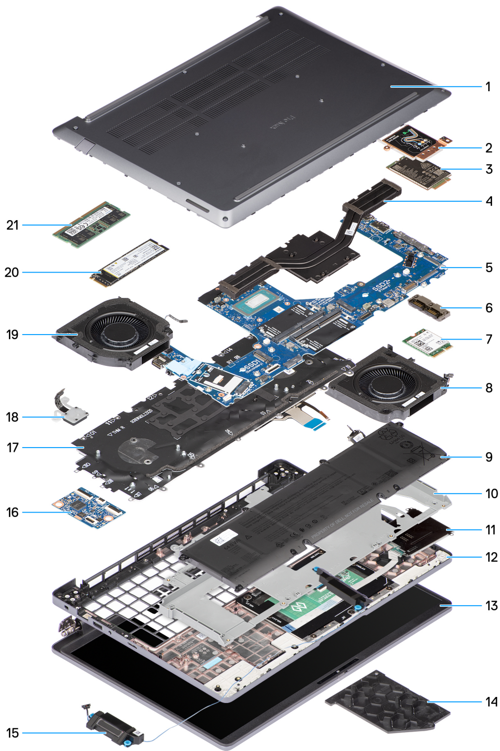
Figur 11. Huvudkomponenter i Dell Pro Max 16 MC16250
