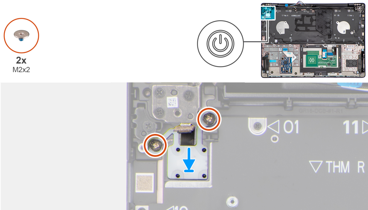
Figur 97. Installera strömbrytaren
