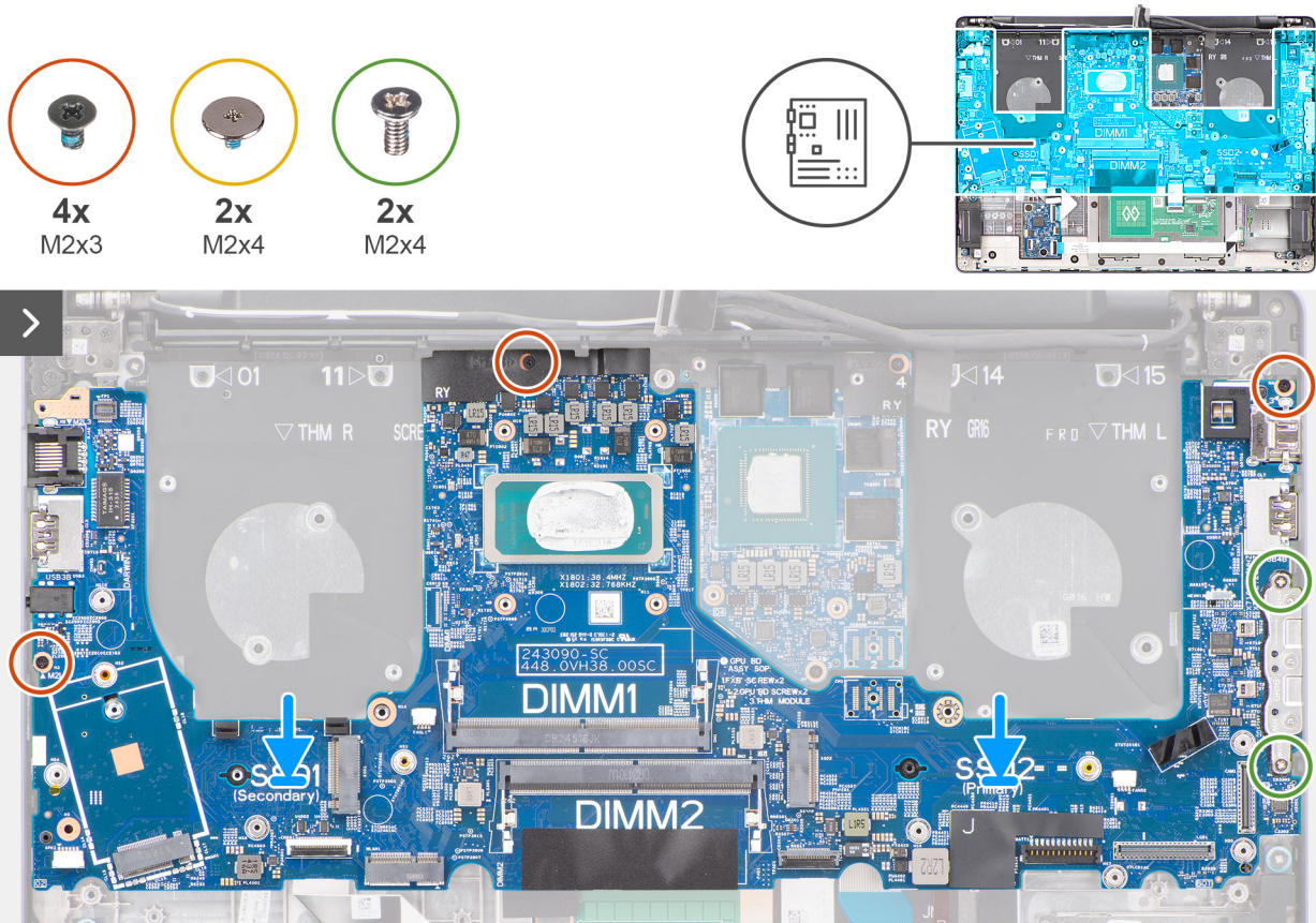
Figur 92. Installera moderkortet
