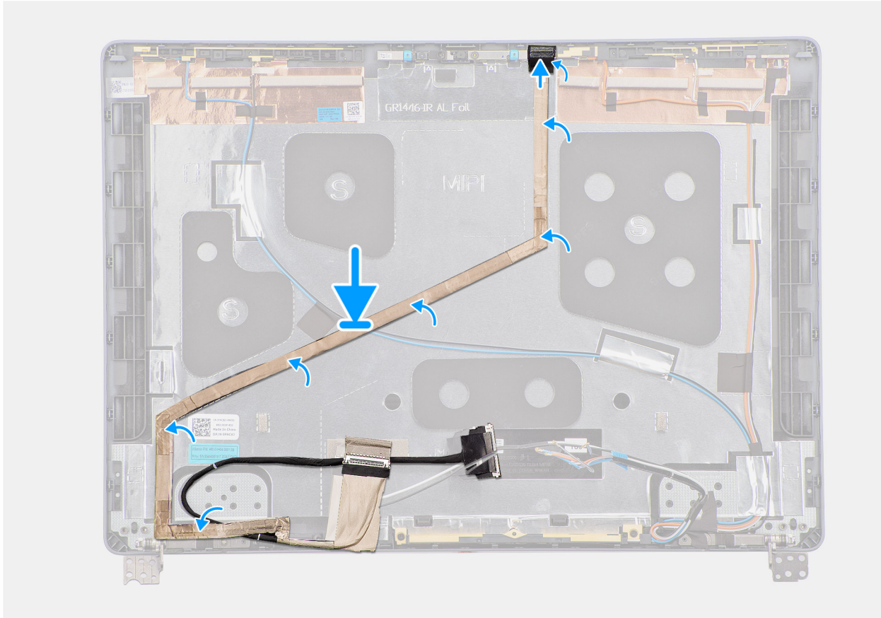
Figur 77. Installera bildskärmskabeln
