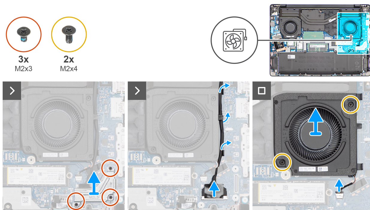
Figur 38. Ta bort den vänstra/videofläkten
