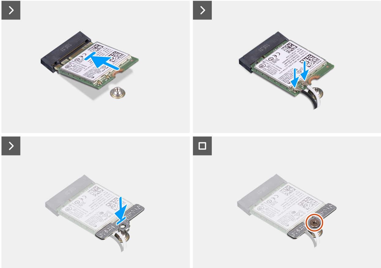
Figur 28. Installera det trådlösa kortet
