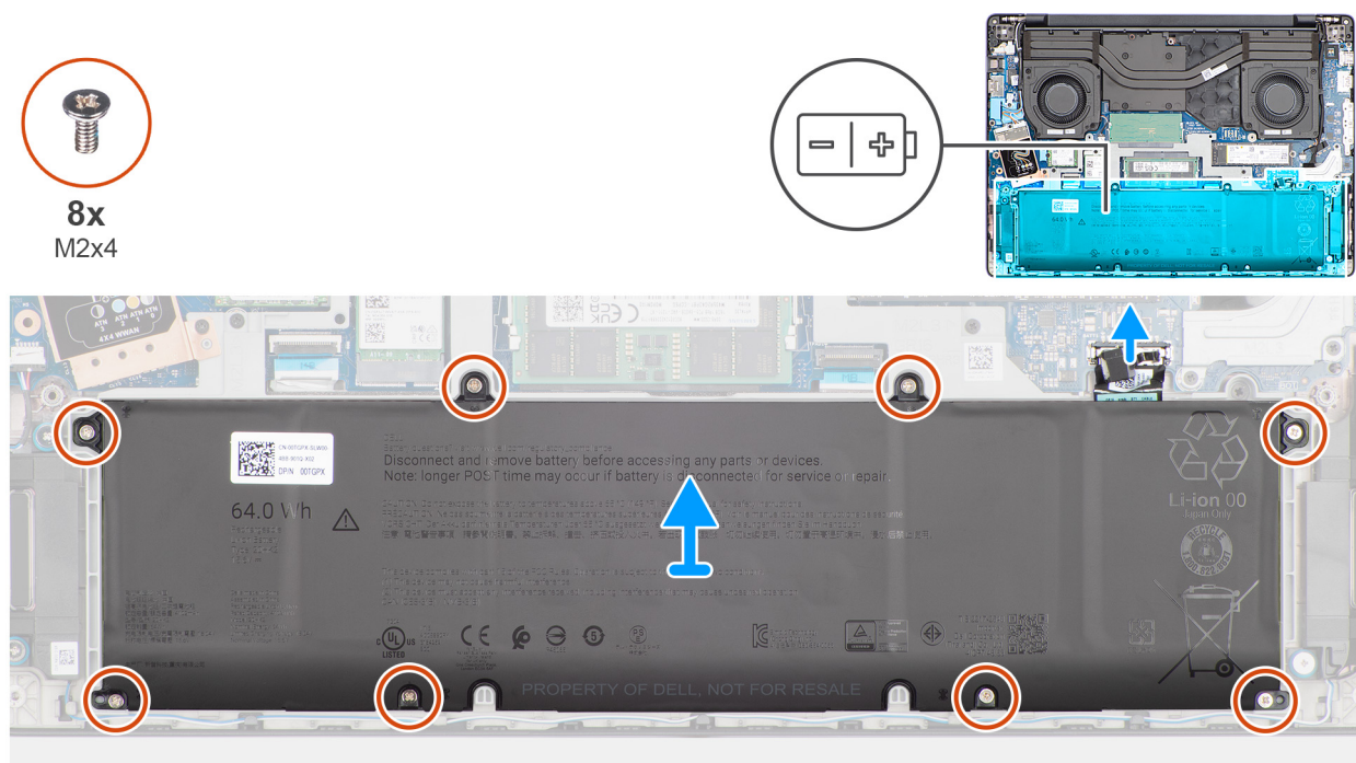
Figur 17. Ta bort batteriet
