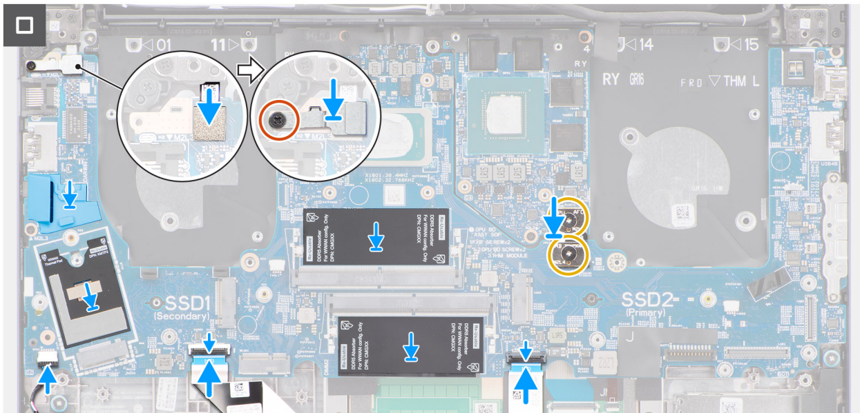
Figur 93. Installera moderkortet
