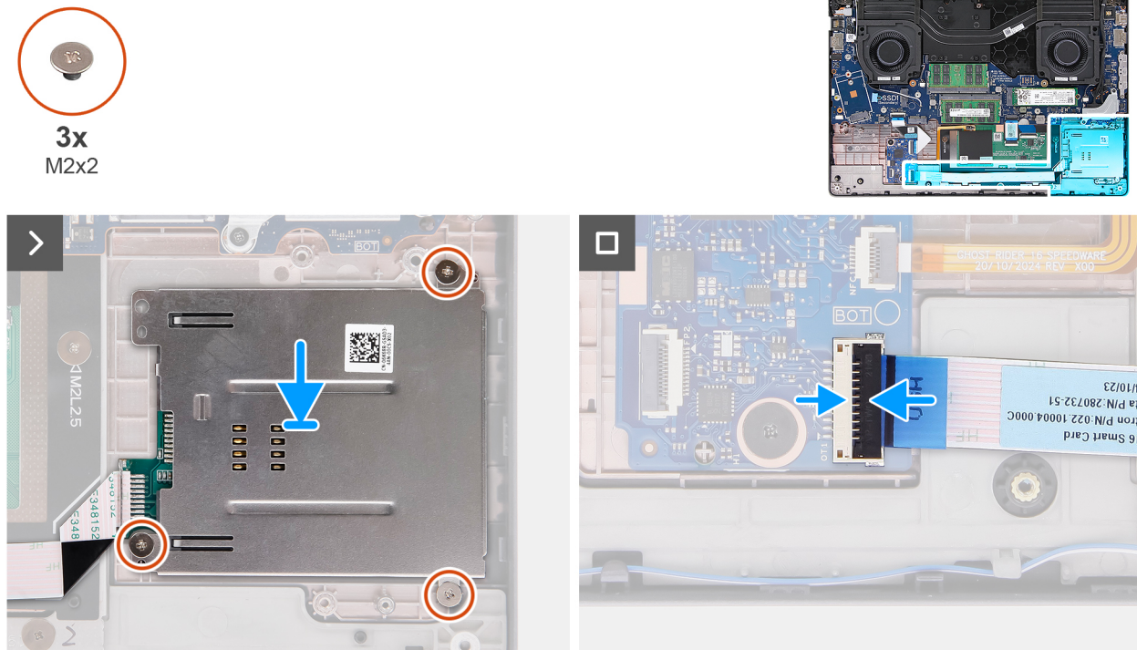
Figur 53. Installera smartkortläsaren
