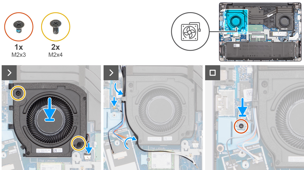
Figur 37. Installera den högra processorfläkten/processorfläkten
