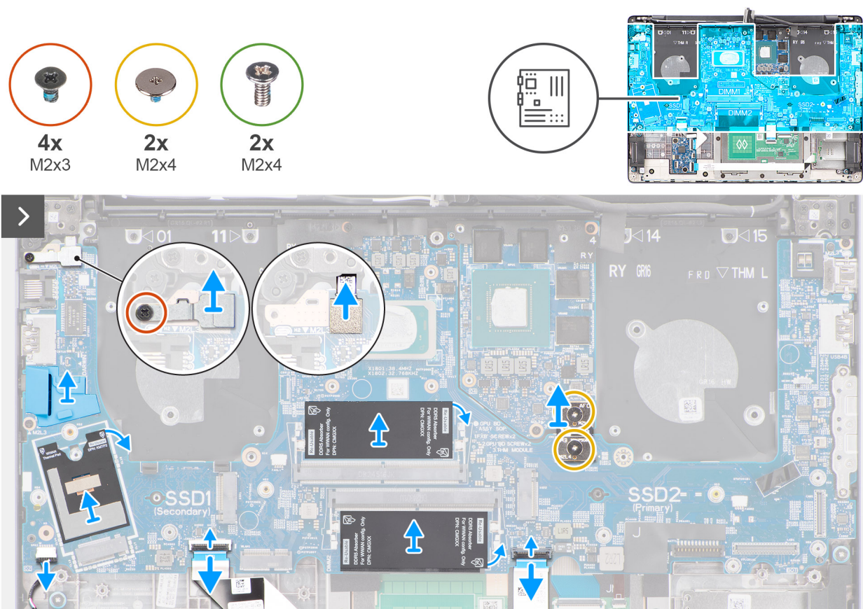
Figur 89. Ta bort systemkort
