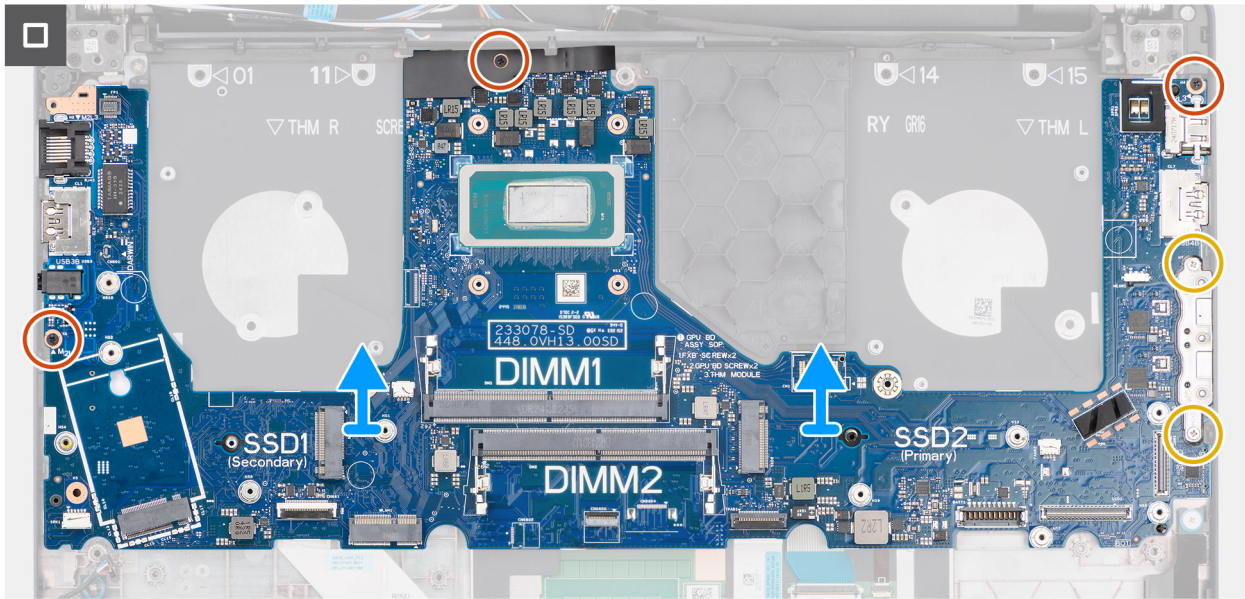
Figur 84. Ta bort systemkort
