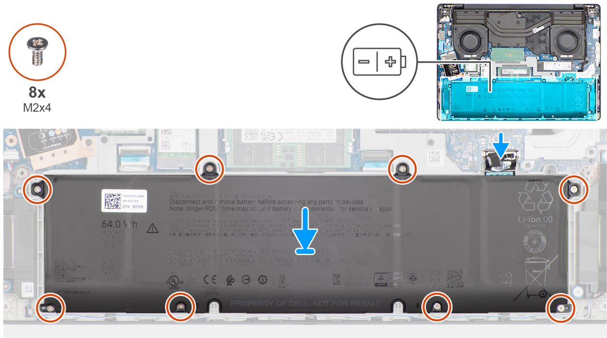
Figur 18. Installera batteriet
