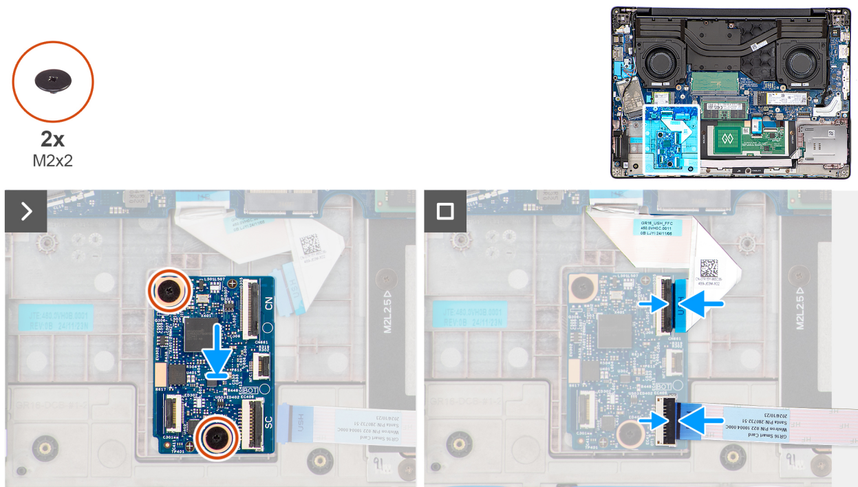
Figur 51. Installera USH-kortet
