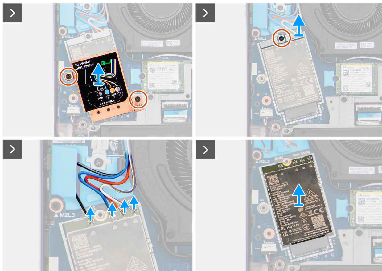
Figur 29. Ta bort WWAN-modulen
