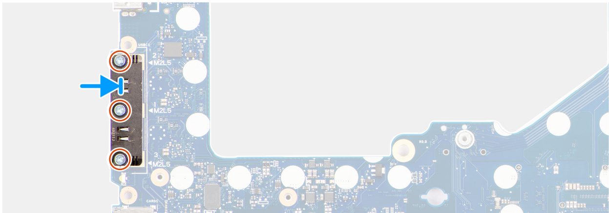
Figur 95. Installera USB Type-C-modulen
