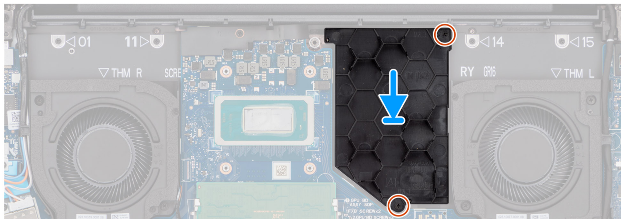
Figur 45. Installera GPU-utfyllnaden
