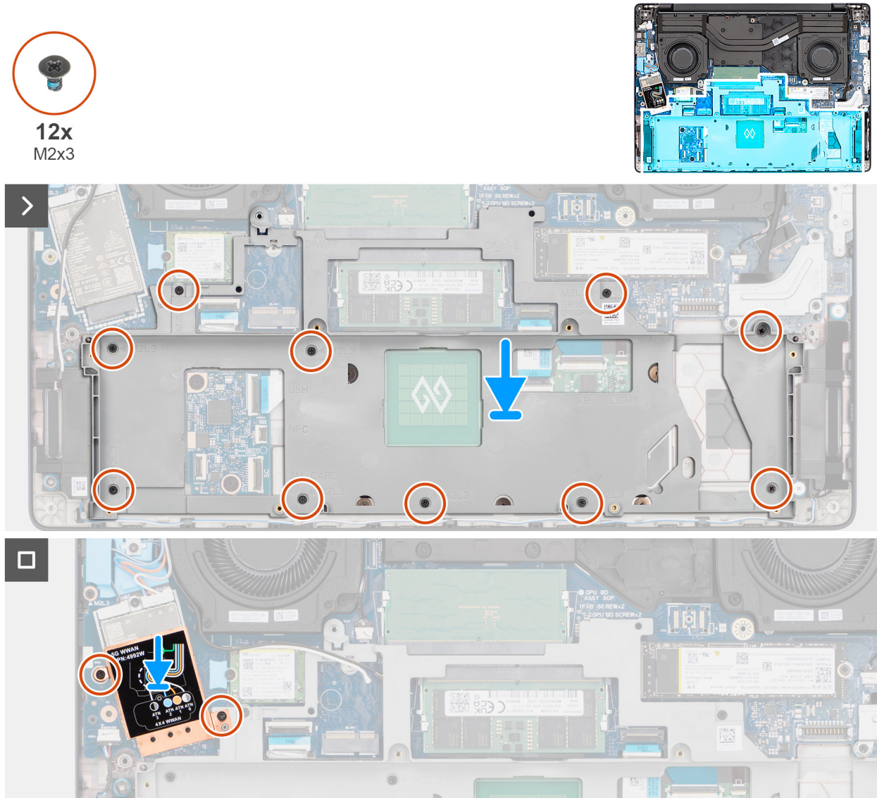
Figur 49. Installera batteriramen
