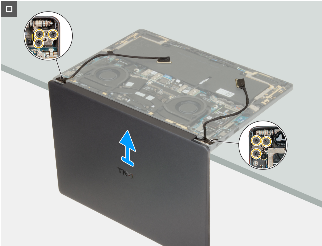
Figur 59. Ta bort bildskärmsenheten
