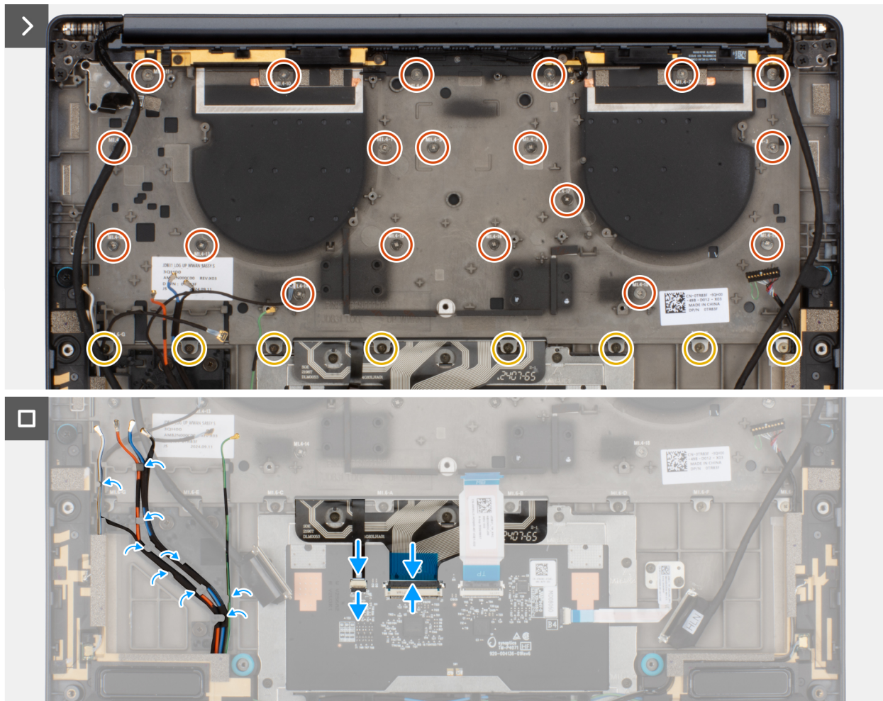
Figur 76. Installera tangentbordsenheten
