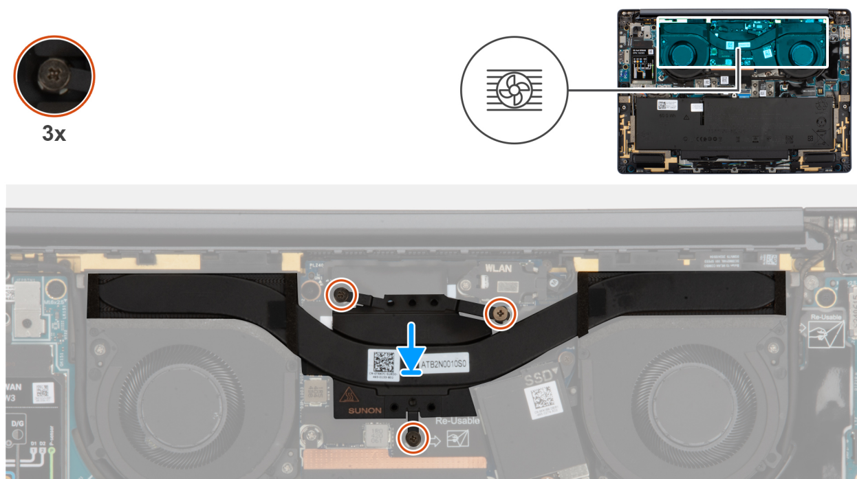
Figur 39. Installera kylflänsen
