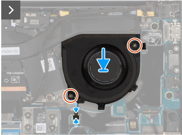
Figur 31. Installera den vänstra fläkten
