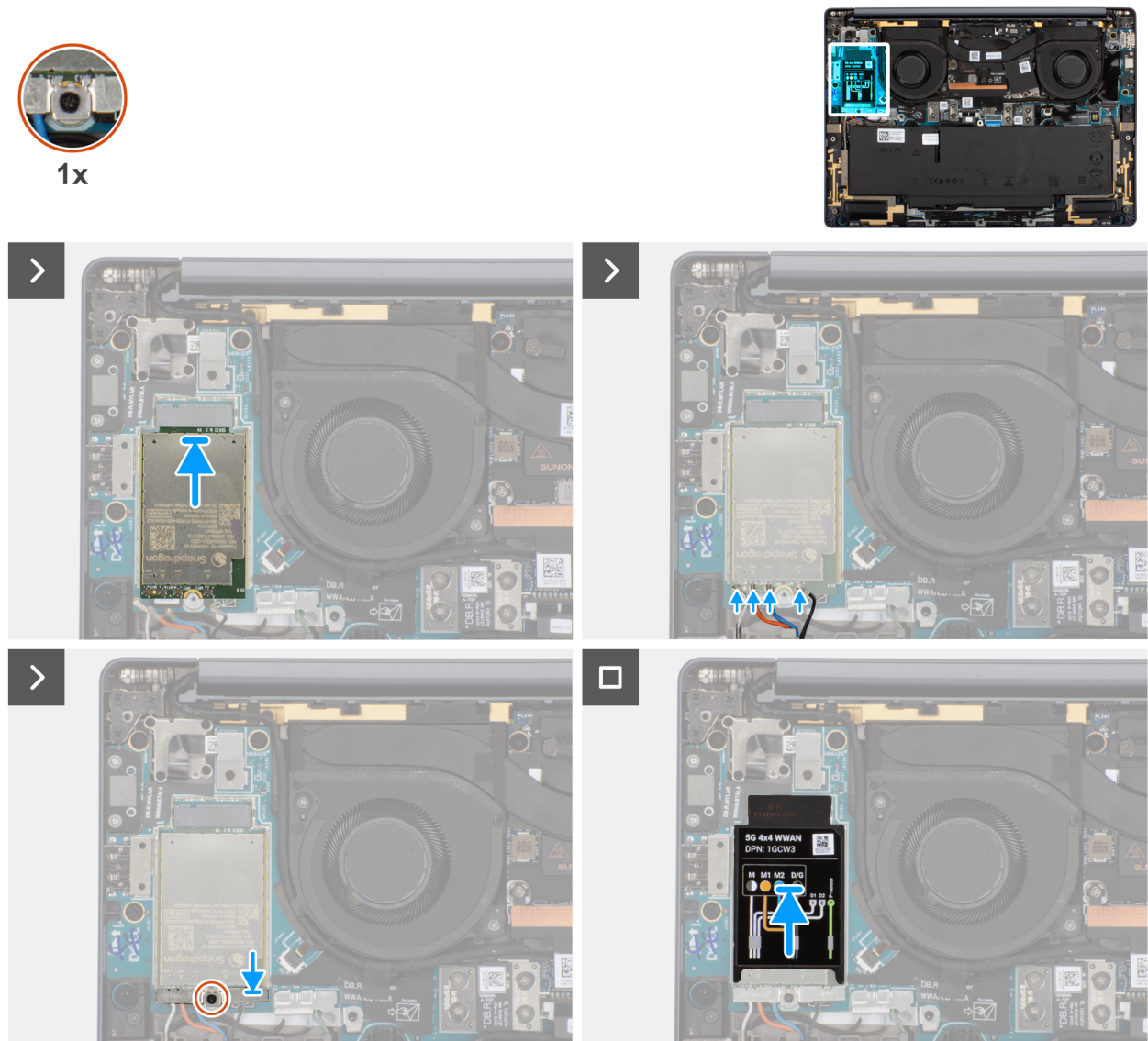
Figur 29. Installera WWAN-kortet
