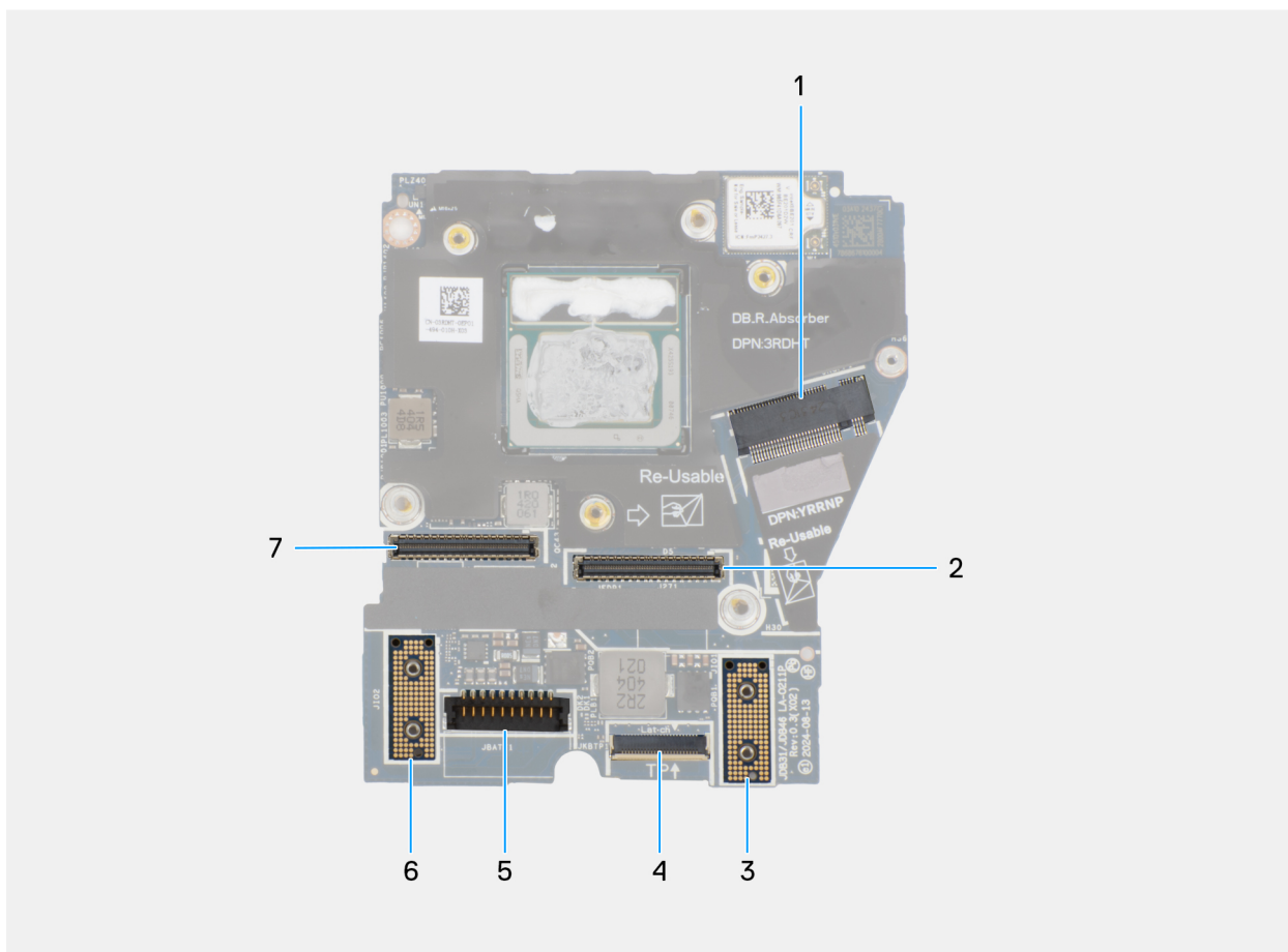
Figur 68. Moderkort med bildtext
