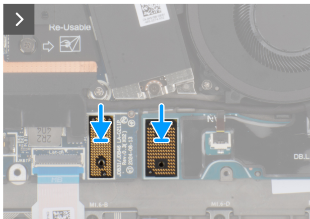
Figur 42. Installera det vänstra I/O-kortet
