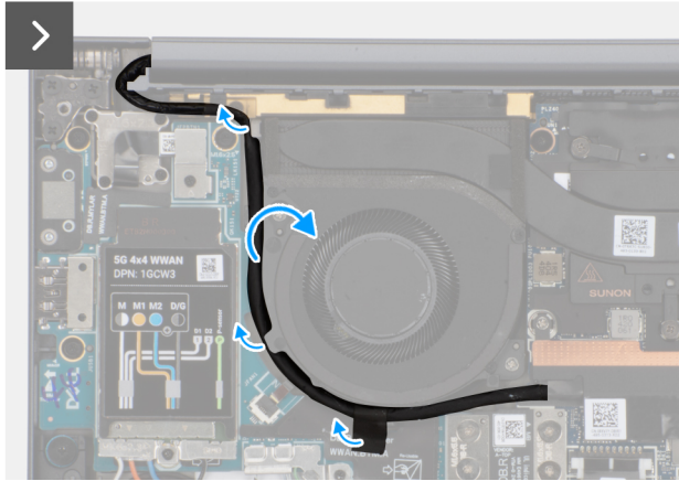
Figur 32. Ta bort den högra fläkten
