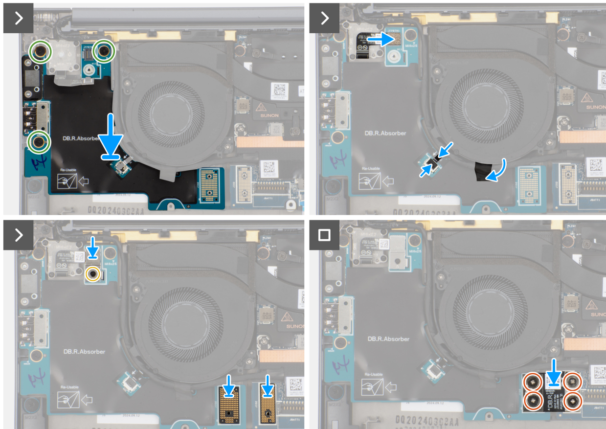
Figur 46. Installera det högra I/O-kortet (utan WWAN-antenner)
