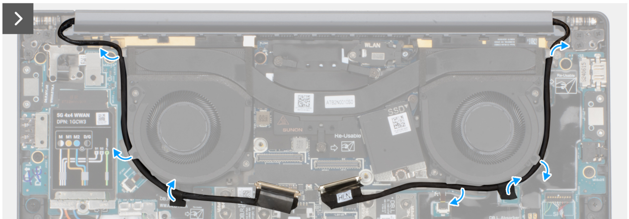
Figur 58. Koppla bort skärm- och kamerakablarna
