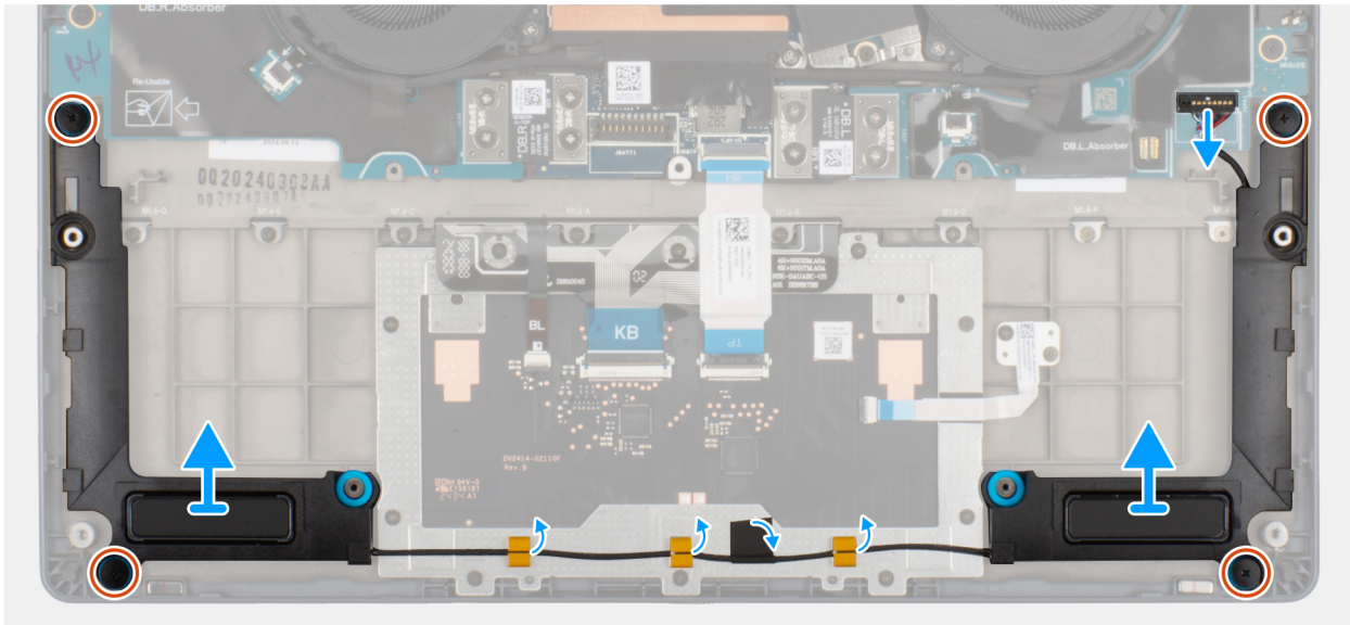
Figur 34. Ta bort högtalarna utan antenn (WLAN-konfiguration)
