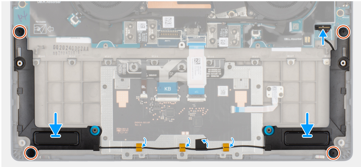
Figur 35. Installera högtalarna (utan WWAN)
