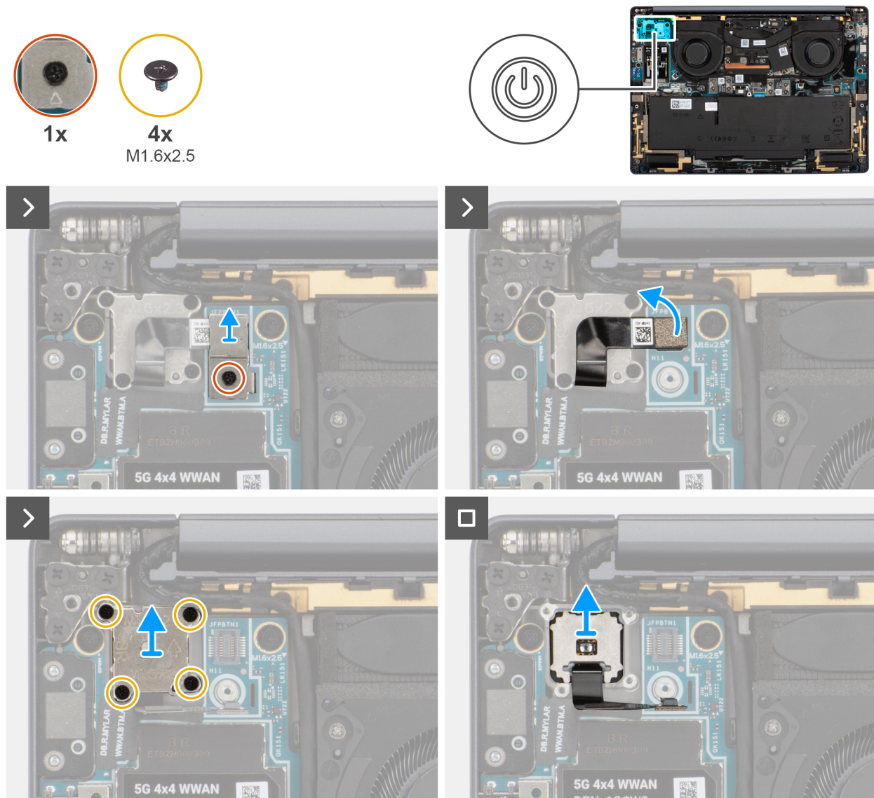
Figur 56. Ta bort strömbrytaren
