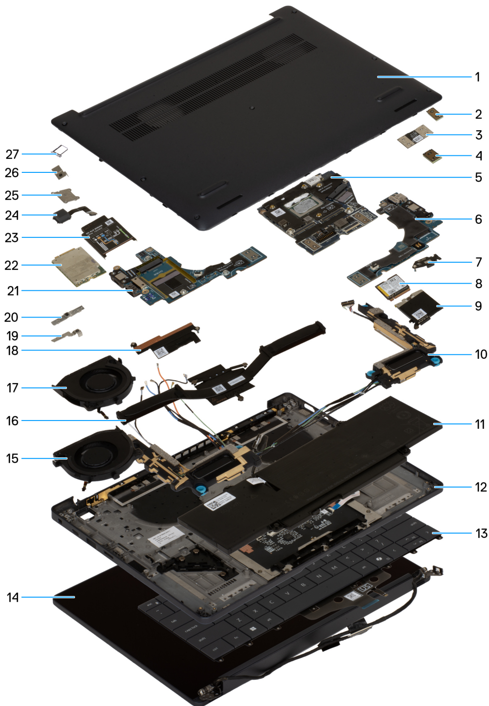
Figur 11. Viktiga komponenter i ditt system/sprängskiss
