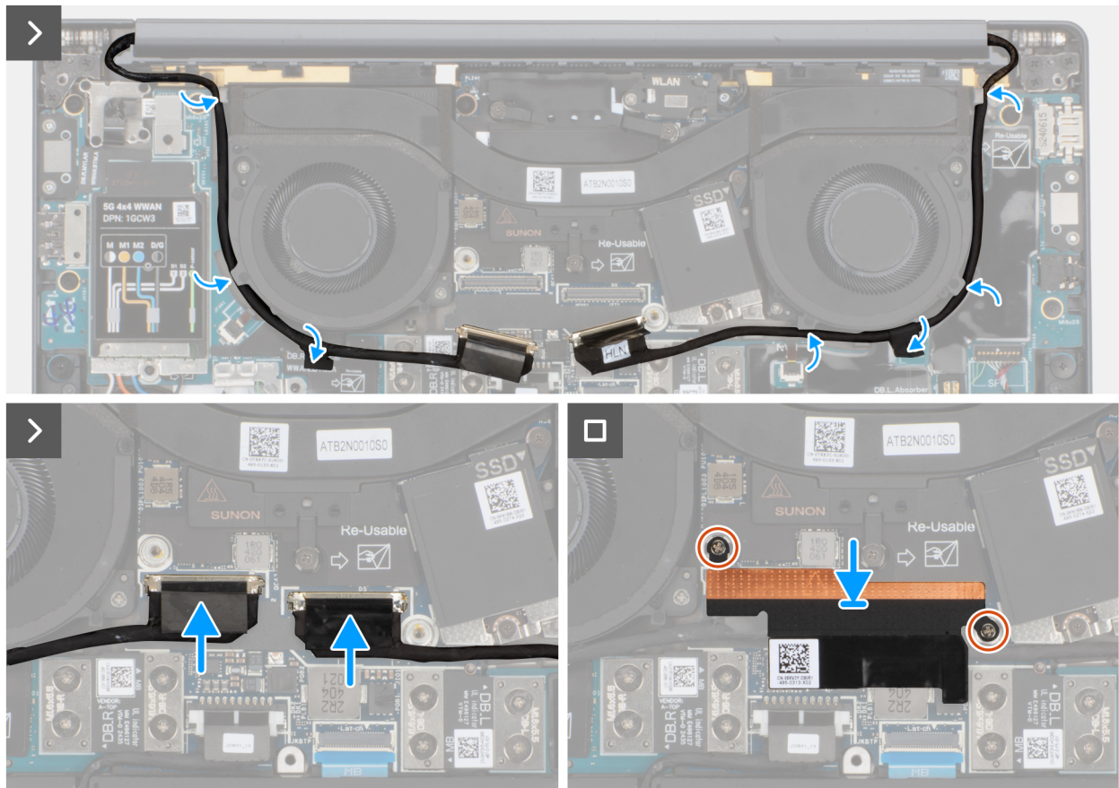
Figur 62. Ansluta skärm- och kamerakablarna
