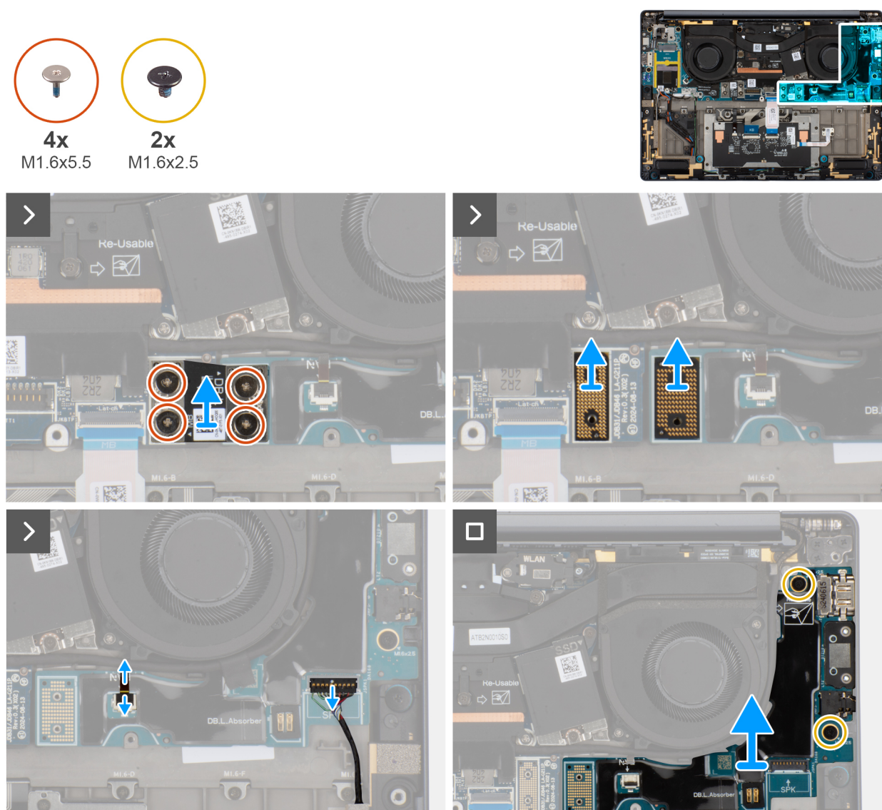
Figur 40. Ta bort det vänstra I/O-kortet
