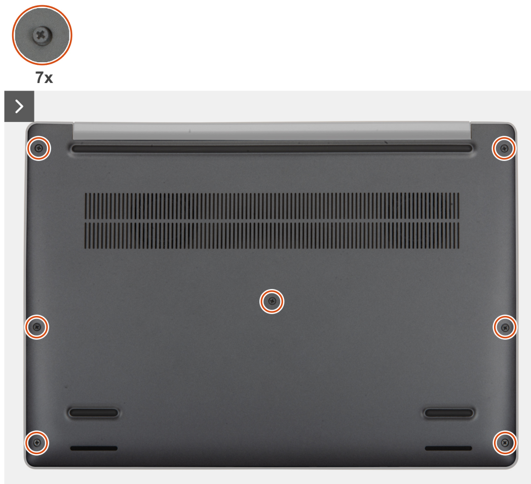
Figur 16. Lossa fästskruvarna
