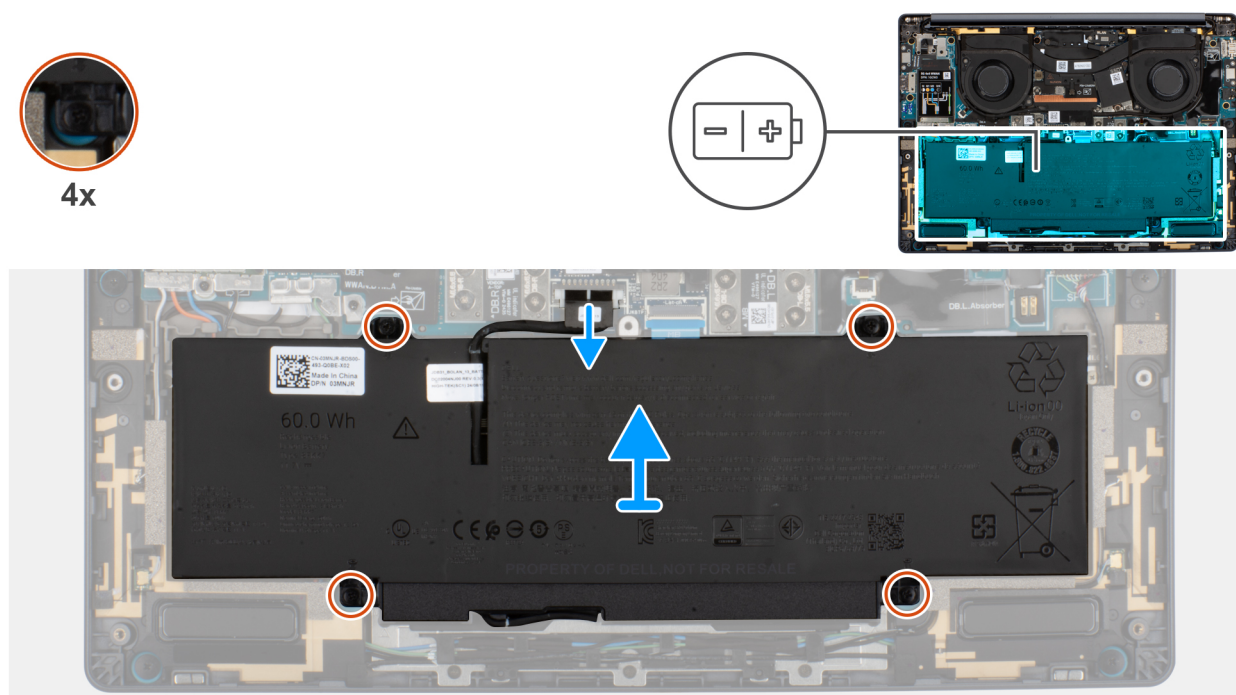
Figur 22. Lossa fästskruvarna
