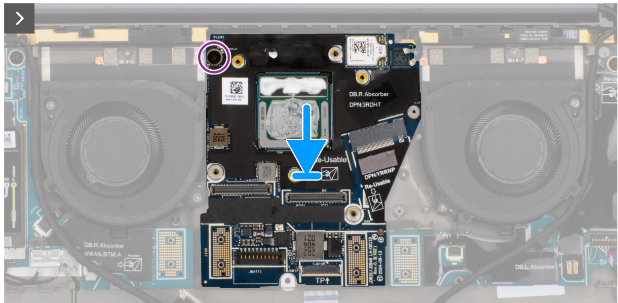
Figur 69. Installera moderkortet
