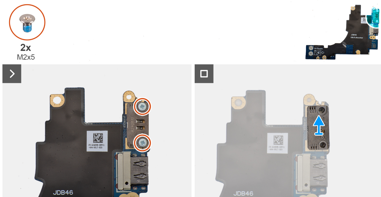
Figur 52. Ta bort den vänstra USB Type-C-modulen
