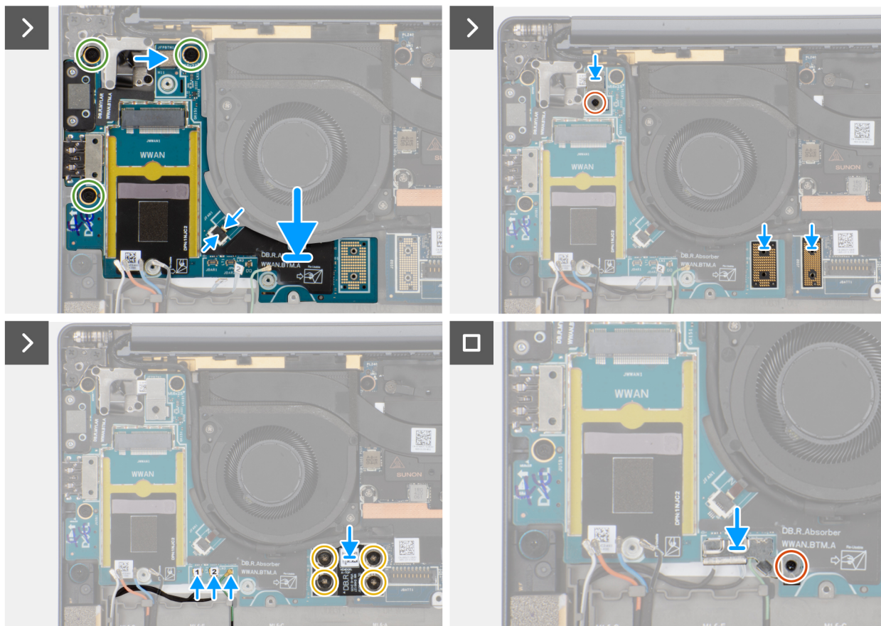
Figur 50. Installera det högra I/O-kortet (med WWAN)
