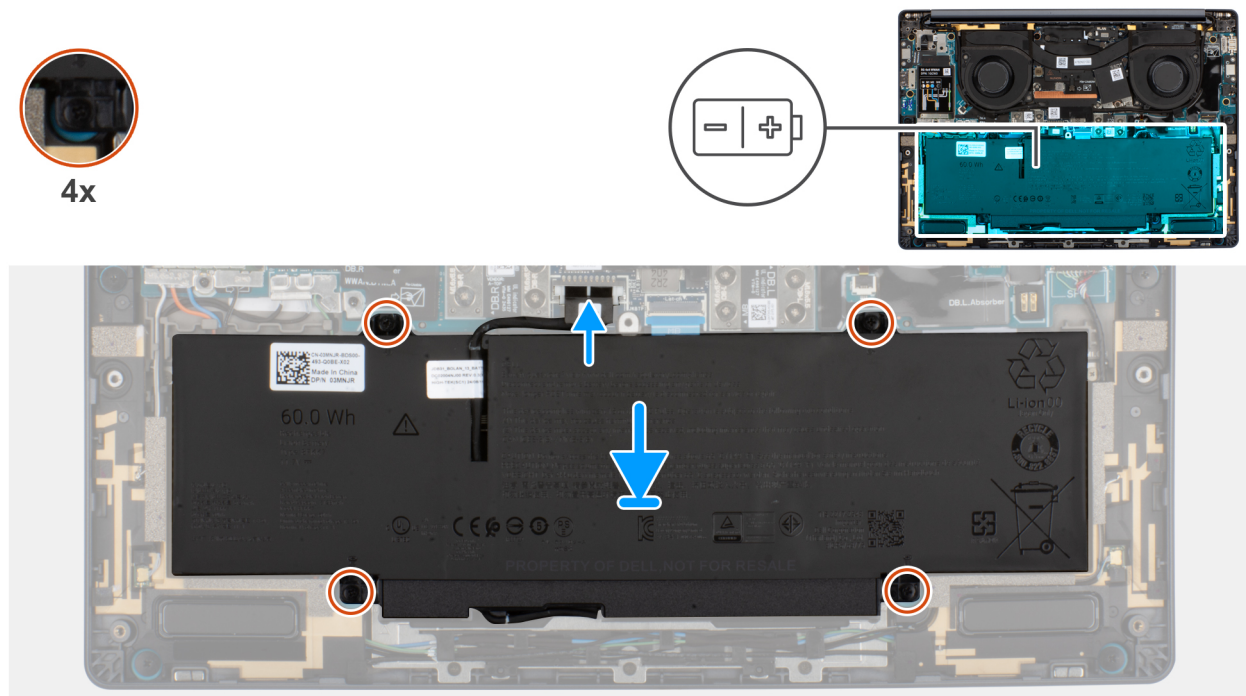
Figur 23. Installera batteriet
