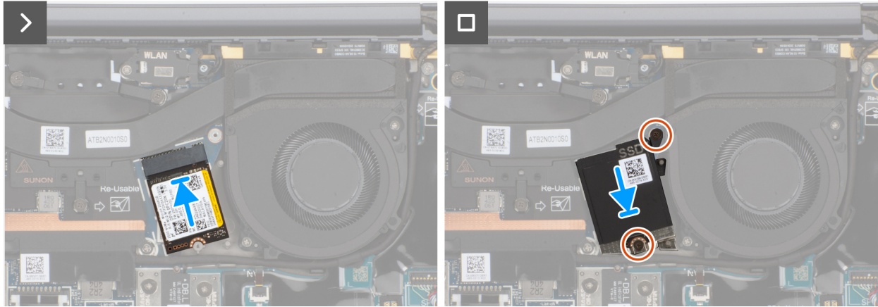
Figur 27. Installera SSD
