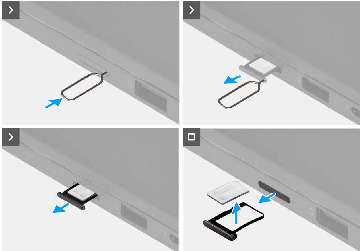
Figur 14. Ta bort nano-SIM-kortet
