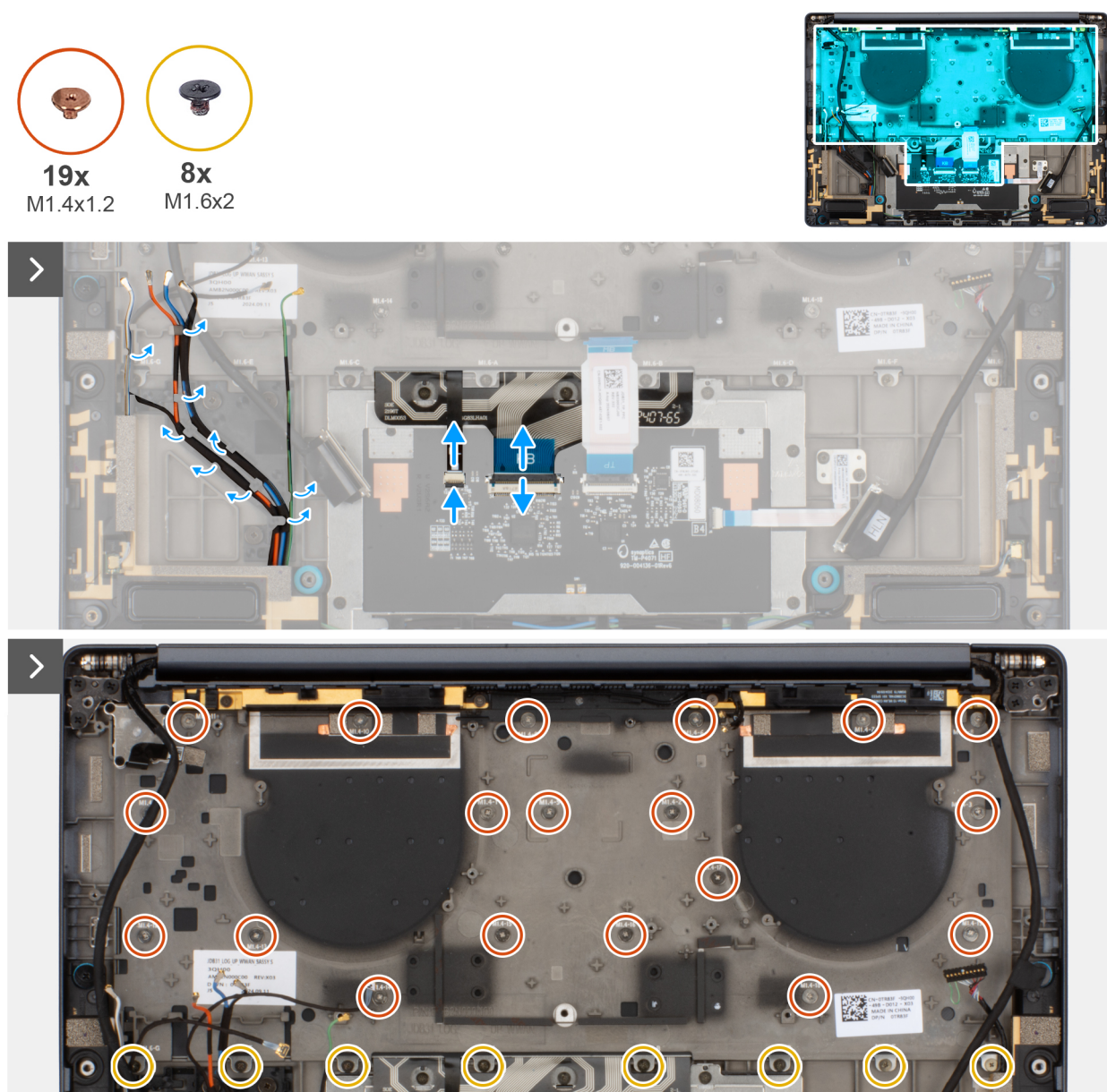
Figur 73. Ta bort tangentbordsenheten
