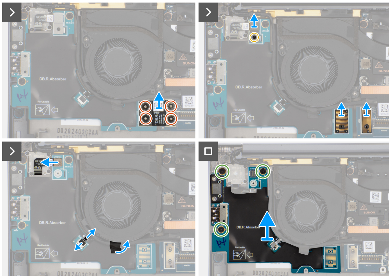
Figur 44. Ta bort det högra I/O-kortet (utan WWAN-antenn)
