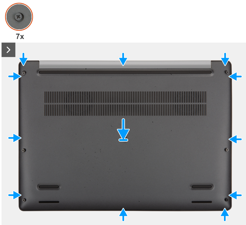
Figur 20. Installera kåpan
