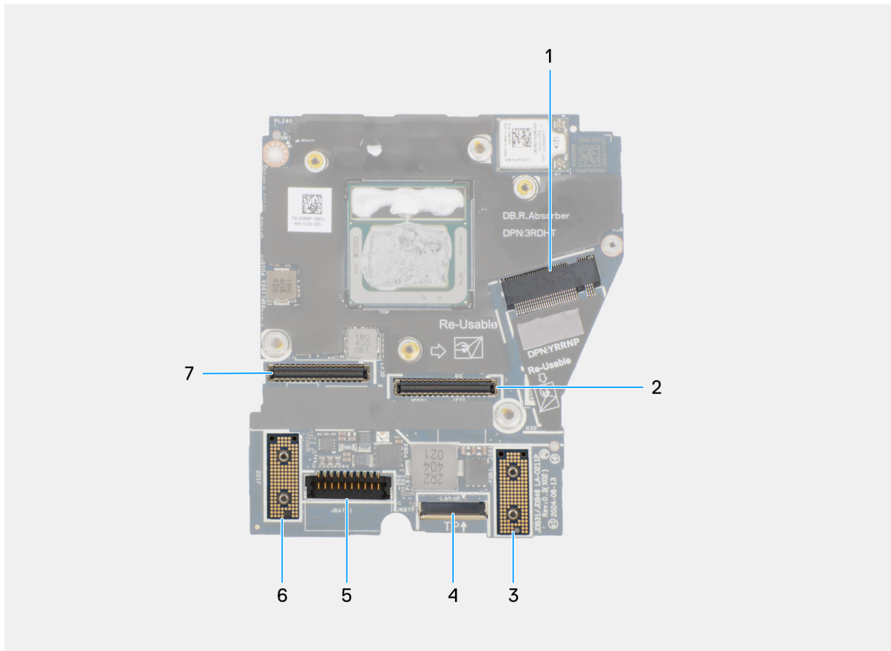
Figur 63. Moderkort med bildtext
