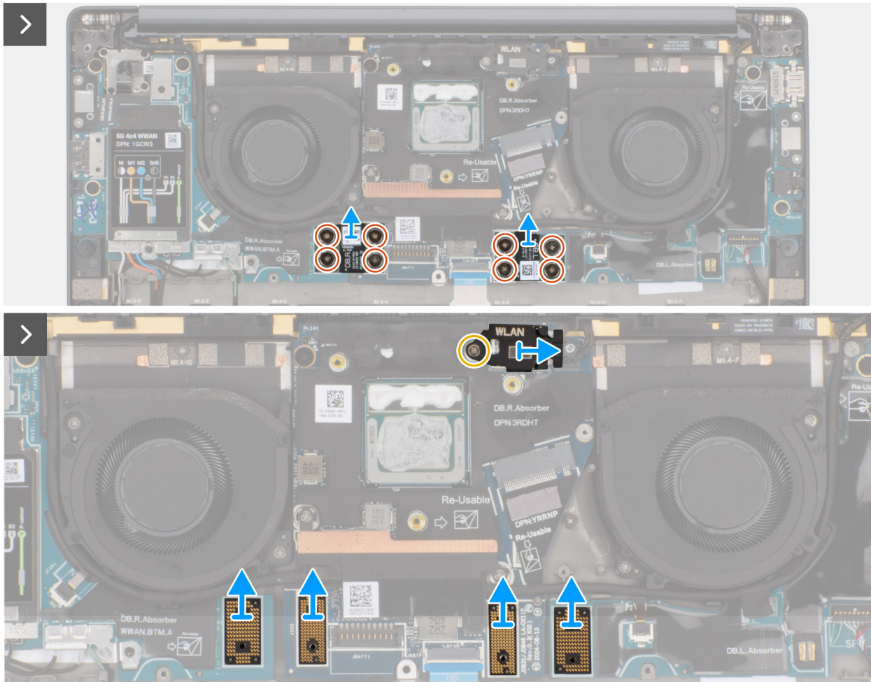
Figur 64. Ta bort moderkortet
