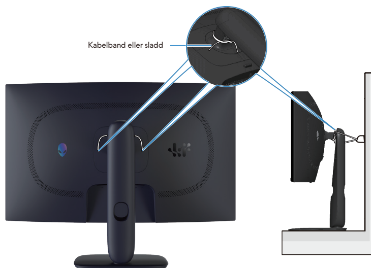
Figure 27. Säkra din skärm
