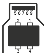
Figure 7. USB-B uppströmsport
