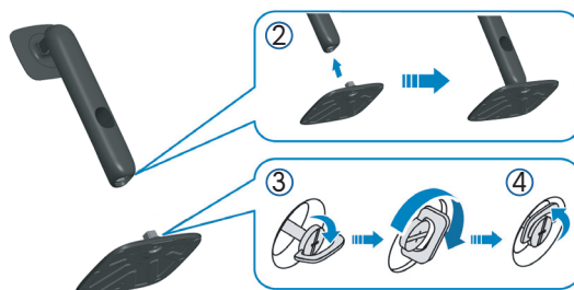
Figure 14. Montera stativets stigdel på stativbasen
