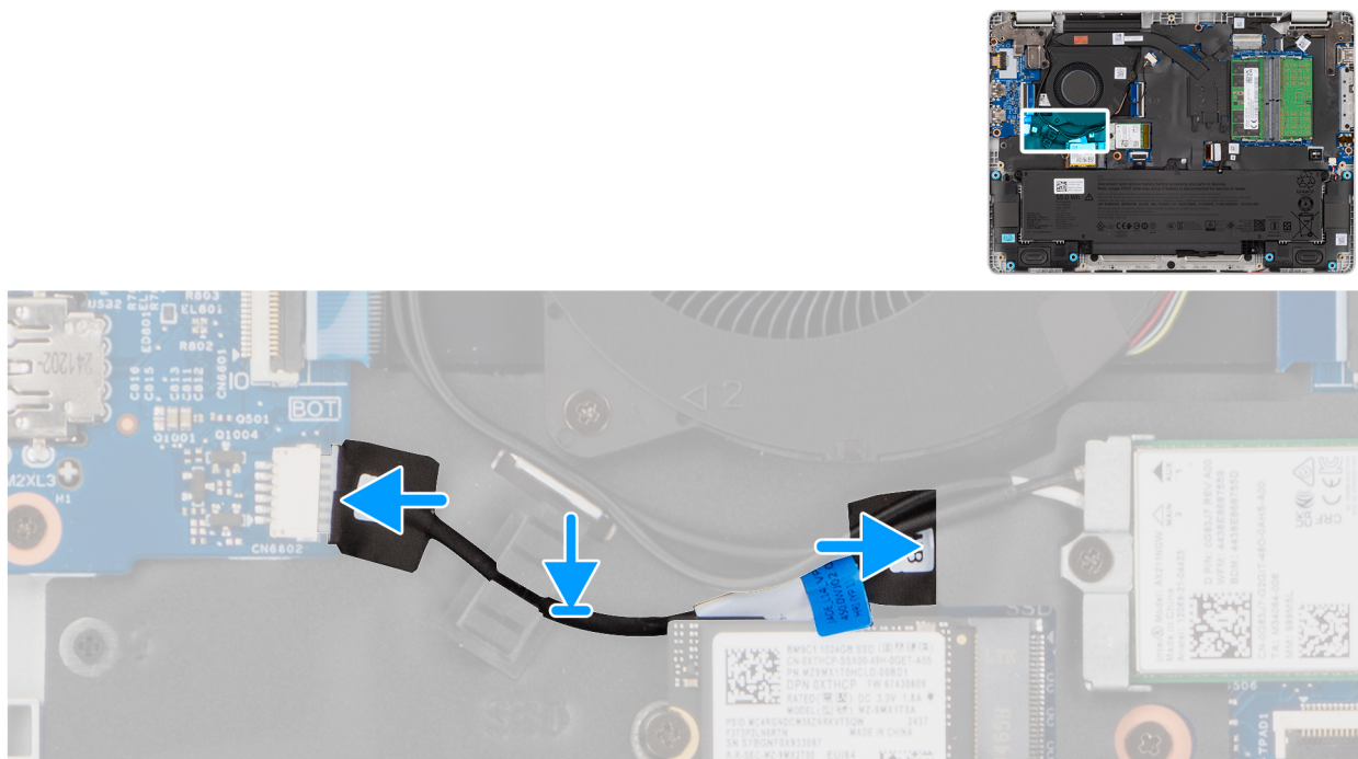
Figur 37. Installera vPro-kabeln
