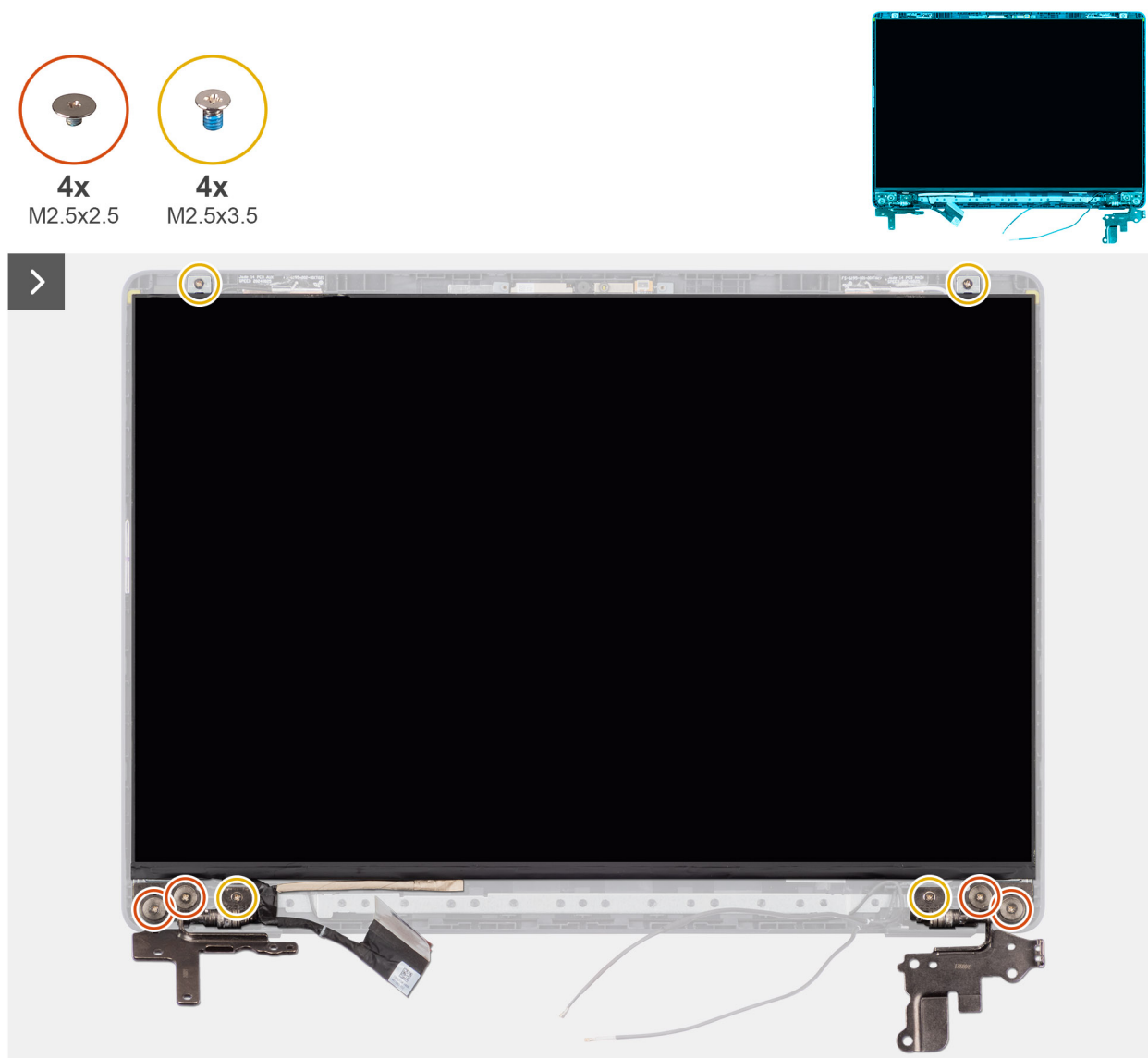
Figur 84. Ta bort bildskärmspanelen
