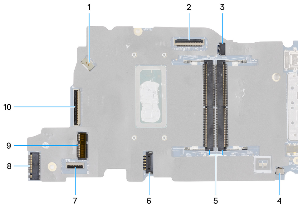
Figur 49. Moderkortets kontakter
