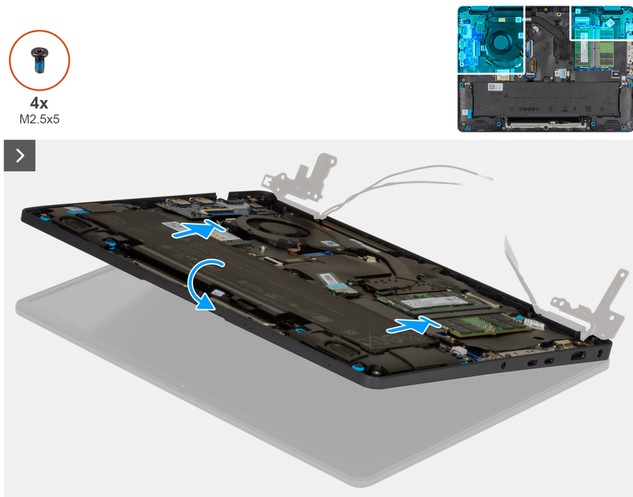
Figur 75. Installera bildskärmsenheten
