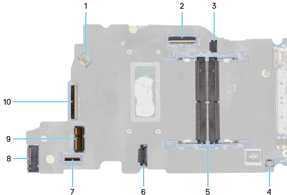
Figur 46. Moderkortets kontakter
