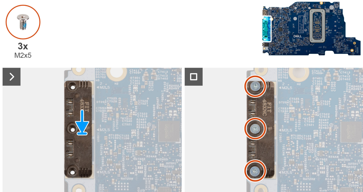
Figur 59. Installera USB Type-C-modulen
