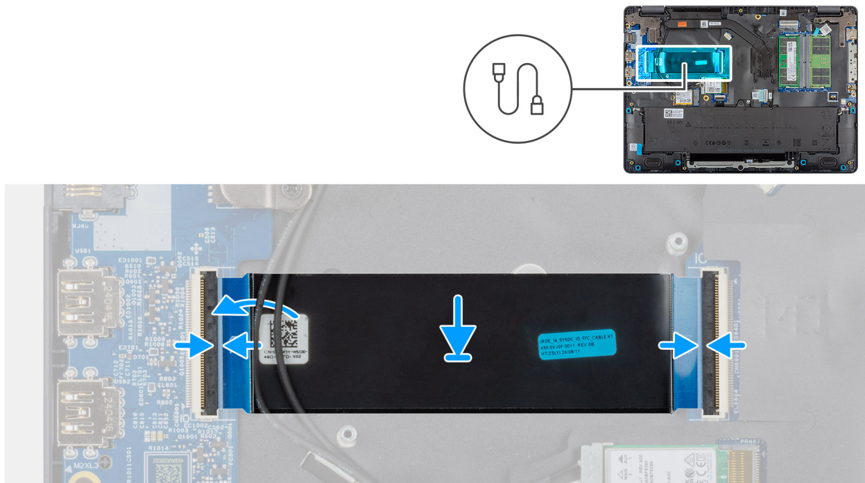
Figur 43. Installera I/O-kortets FPC-kabel
