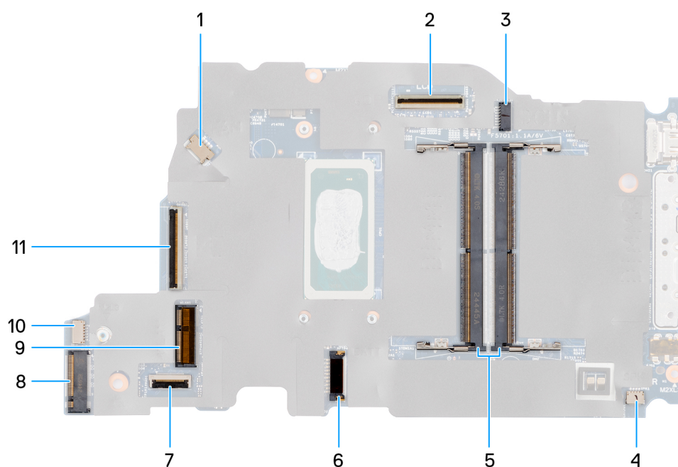
Figur 52. Moderkortets kontakter
