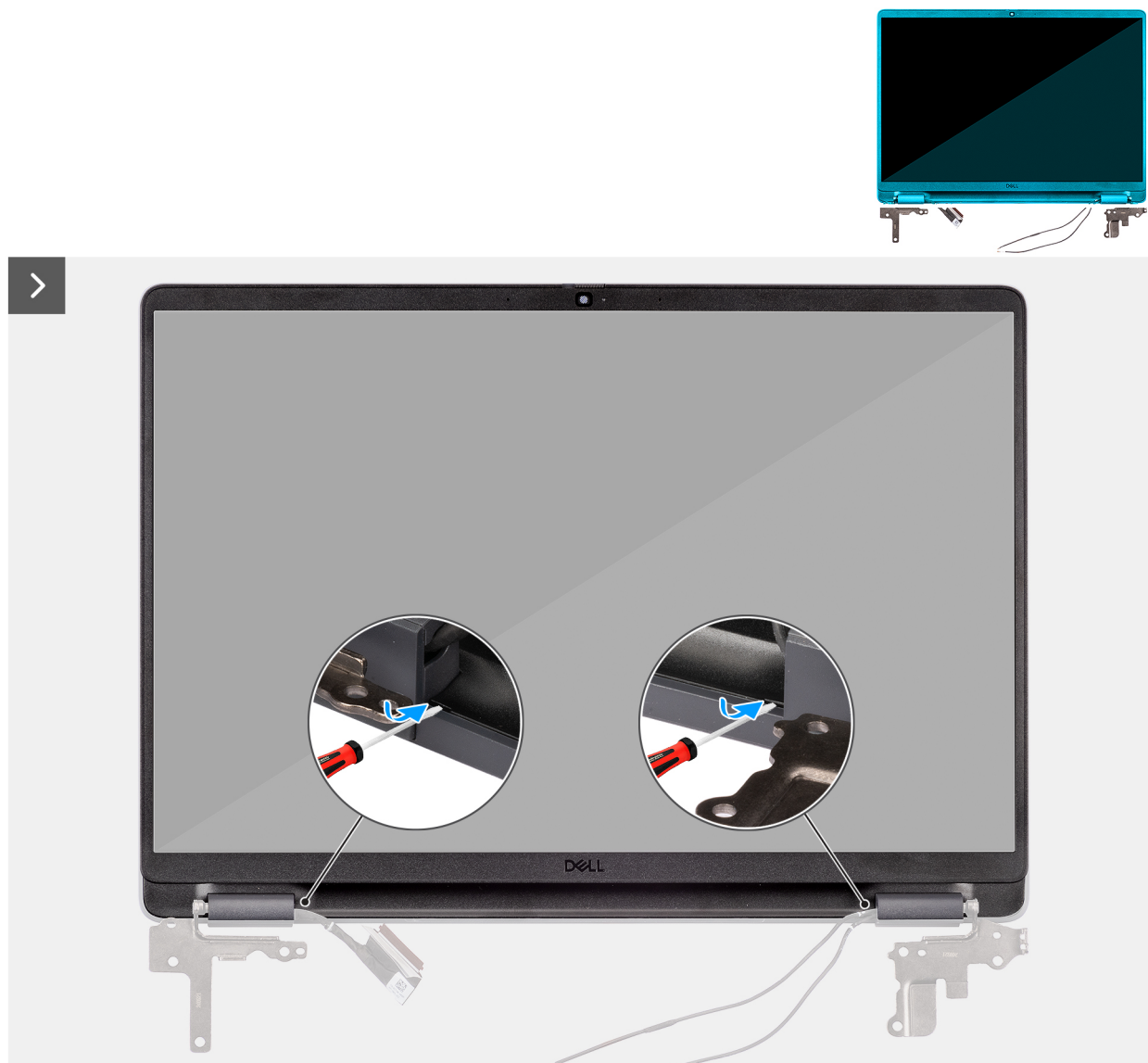
Figur 77. Ta bort bildskärmsramen
