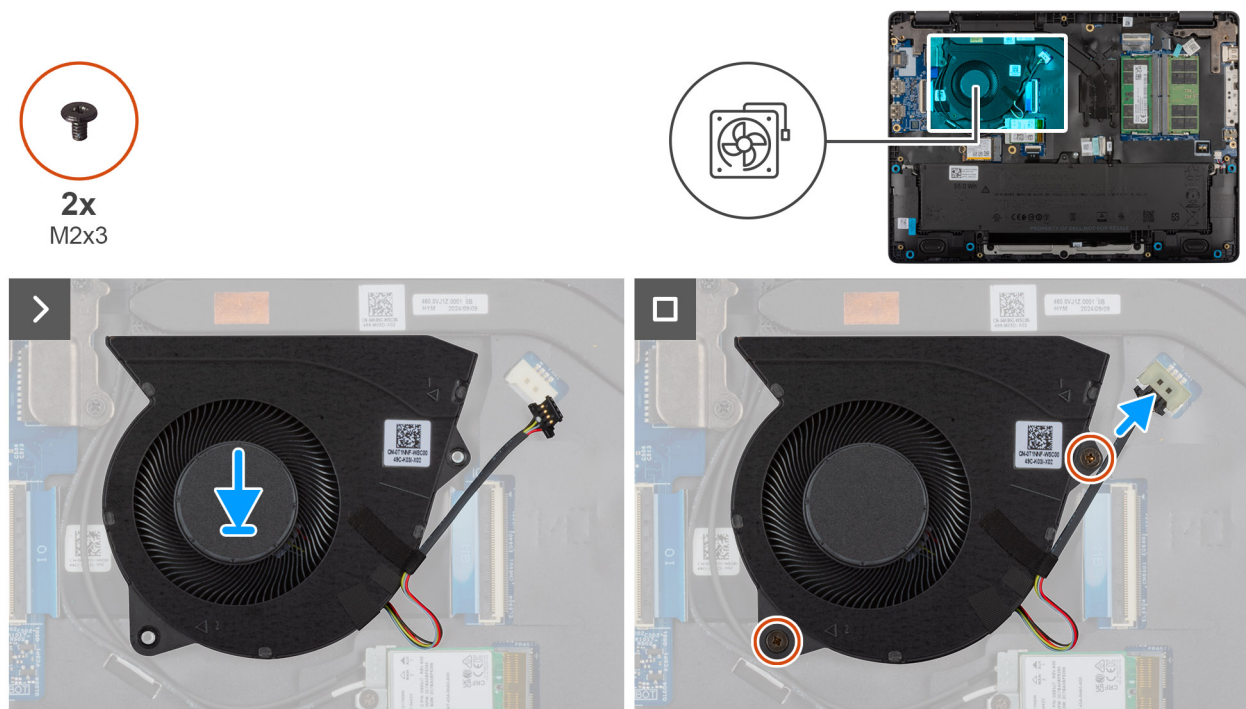
Figur 31. Installera fläkten
