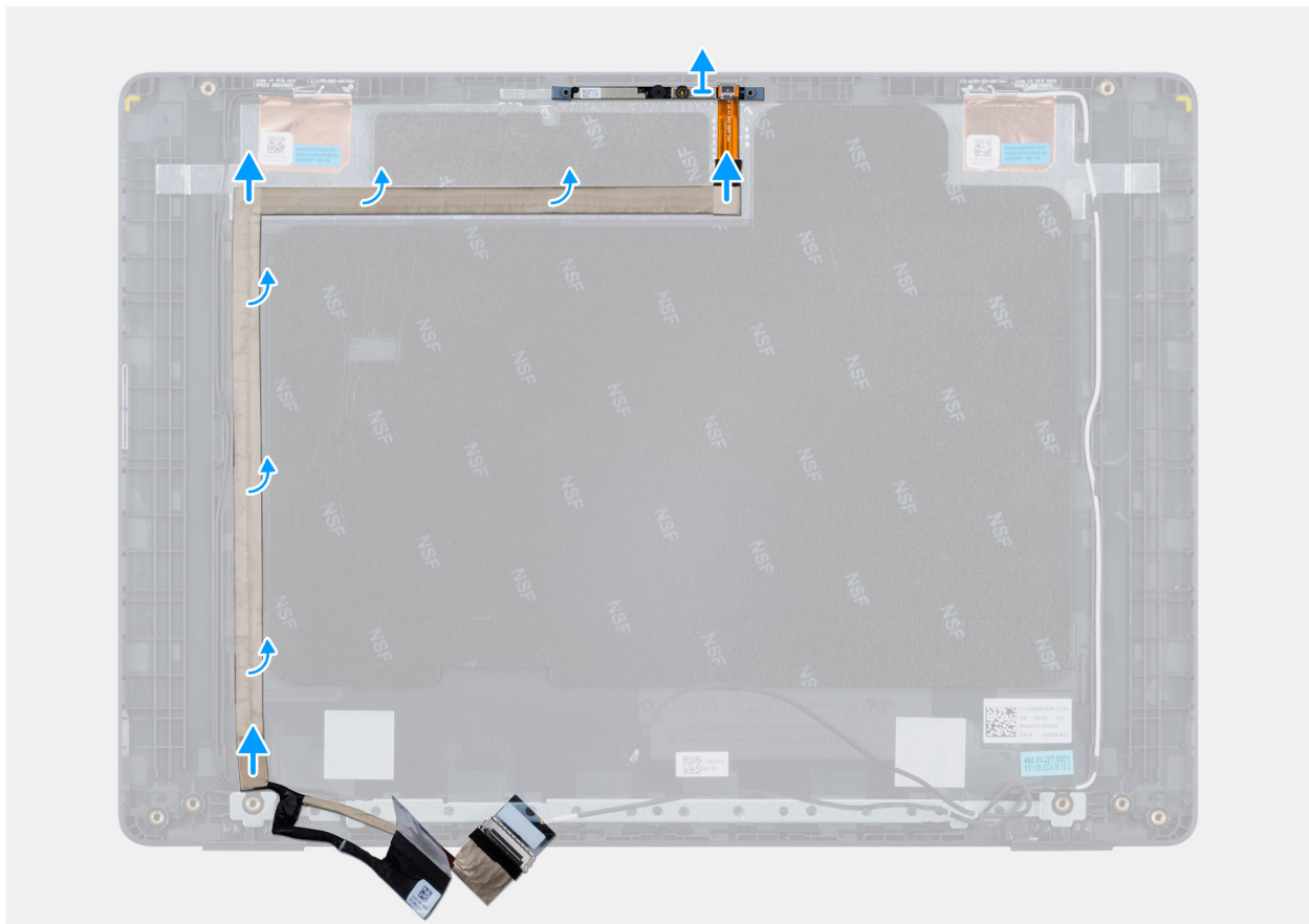
Figur 94. Ta bort eDP-kabeln
