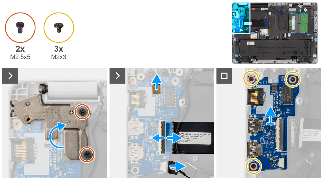
Figur 40. Ta bort I/O-kortet
