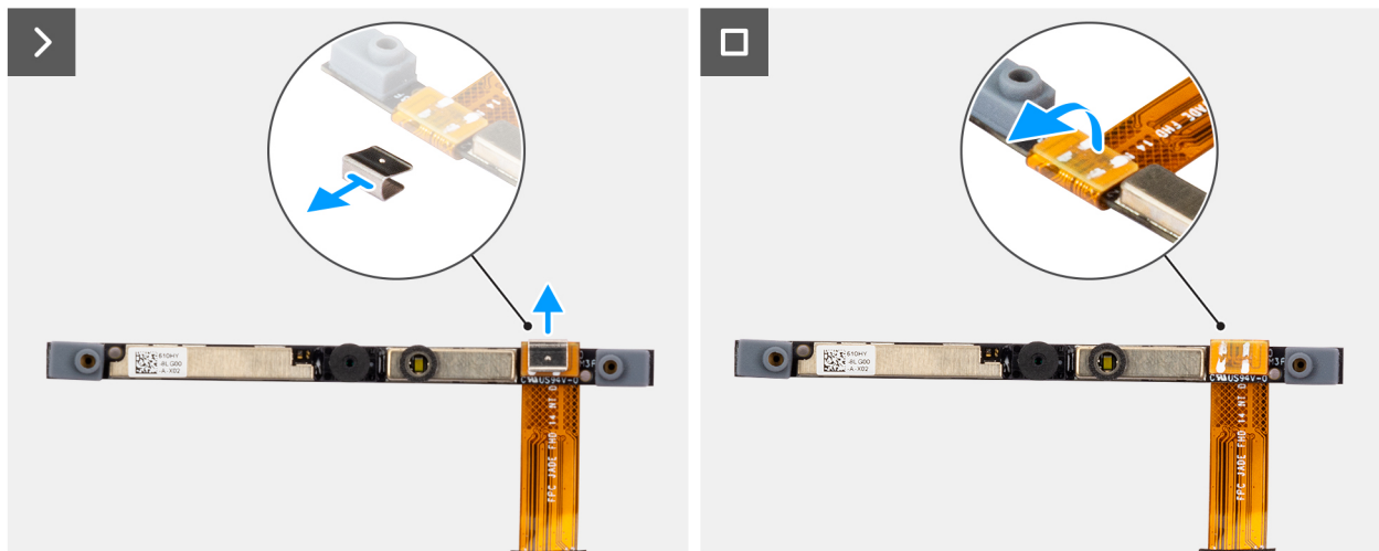
Figur 92. Ta bort kameran
