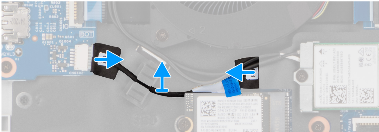
Figur 36. Ta bort vPro-kabeln
