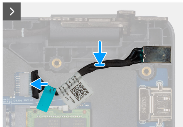
Figur 33. Installera nätaggregatsporten
