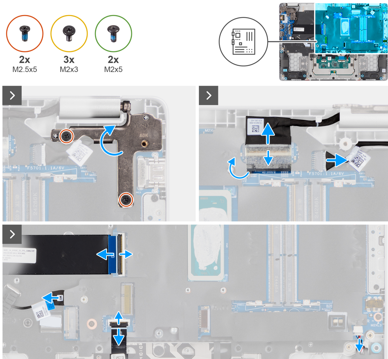
Figur 53. Ta bort moderkortet
