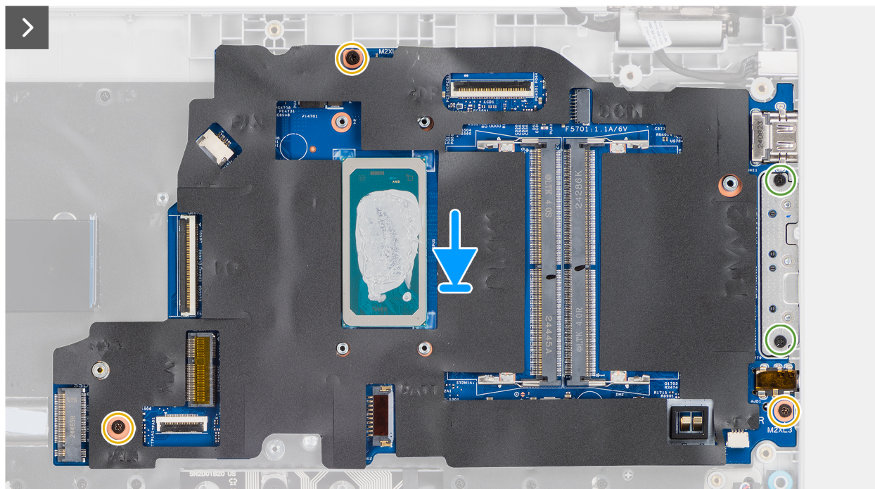
Figur 56. Installera moderkortet
